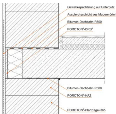
Deckenaufleger: Anschluss an Außenwand mit Deckenrandschale POROTON® DRS® und Höhenausgleichsziegel POROTON® HAZ
