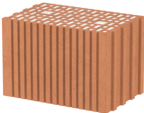
POROTON®-Kimmziegel mit integrierter Perlitedämmung
