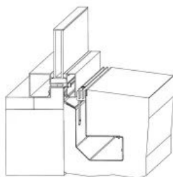
Fassadenschlitzrinne für tiefer liegende Glasfassade
