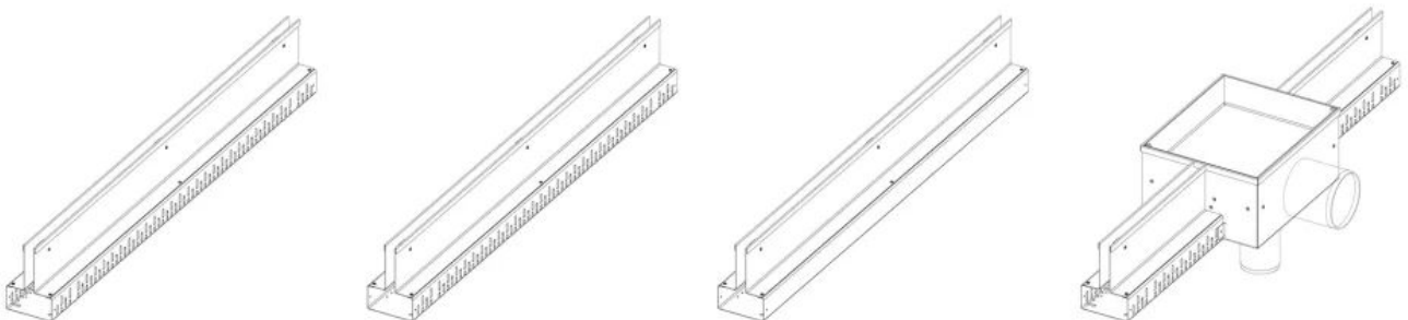
Fassadenschlitzrinne FSR in symmetrischer Ausführung
