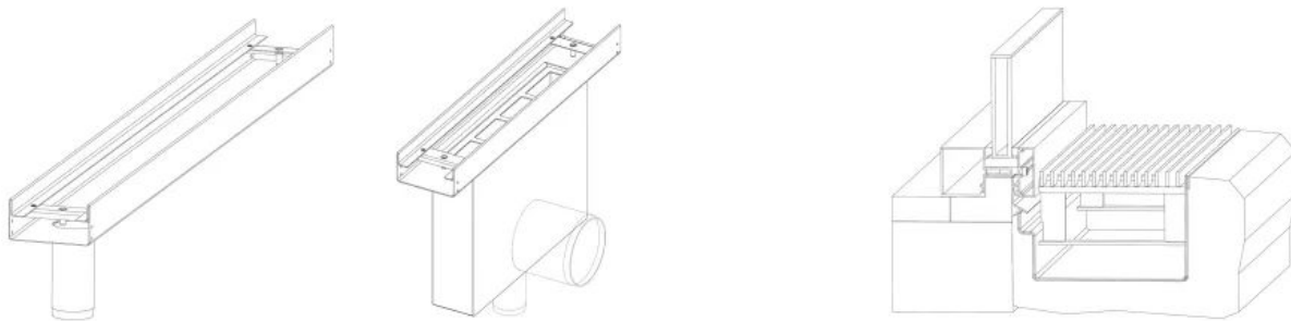
Ablaufvarianten Fassadenkastenrinne FKR
