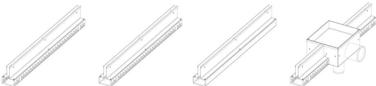
Fassadenschlitzrinne FSR in symmetrischer Ausführung
