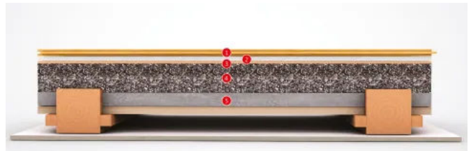
Schwimmender Trockenestrich auf Holzbalkendecke mit schwerer Auffüllung
