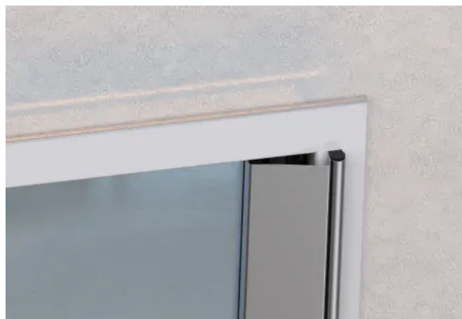
Die Schutzprofile BSG1/BSG2 decken die Bandseite vollständig ab.
