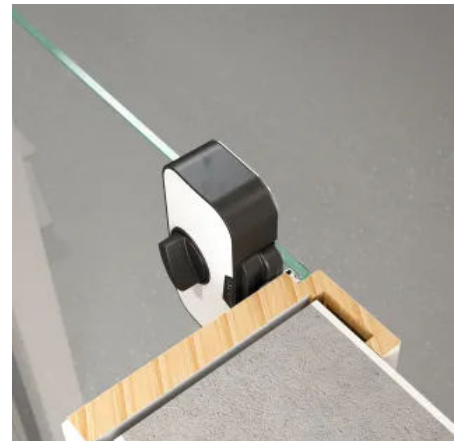
HS-25 Glas: für Glastürmontage mit Spezialklebeband
