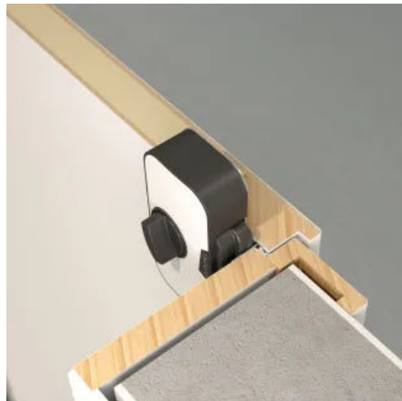
HS-25 einseitig: einfach und effektiv, kein Durchbohren notwendig
