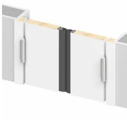
SwingGUARD S sichert Pendeltüren, Karusselltüren und Schiebetüren.
