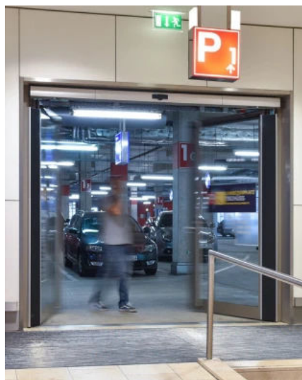
Athmer Fingerschutz® sichert automatische Türen über ihre gesamte Höhe.
