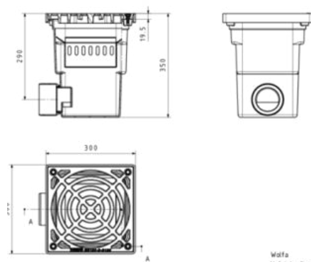
WOLFA Hofeinlaufkasten, Abmessungen
