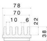
AquaStop Mini, 78 x 38 mm
