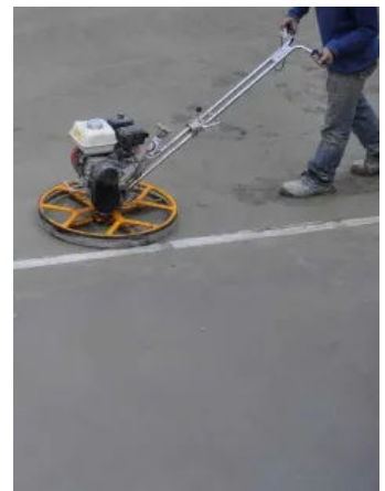
Flügelglätten des Betons bei eingebauter AquaStop Rinne.
