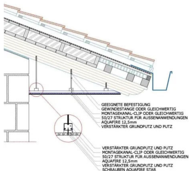
Unterdecke im Außenbereich mit AQUAFIRE-Bekleidung
