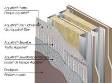
Montagebeispiel für Aquafire Außenanwendung
