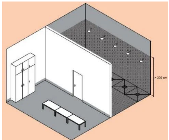
Einsatzbeispiel Verlegeuntergrund für Fliesen in Reihenduschanlage
