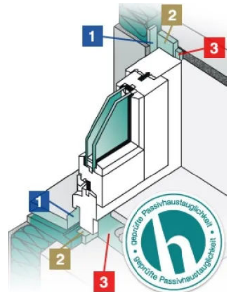
1. Wetterschutzebene, 2. Funktionsebene, 3. Innere Ebene
