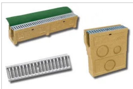
NW 100 Entwässerung für rechteckigen Kunstrasen-Sportplatz
