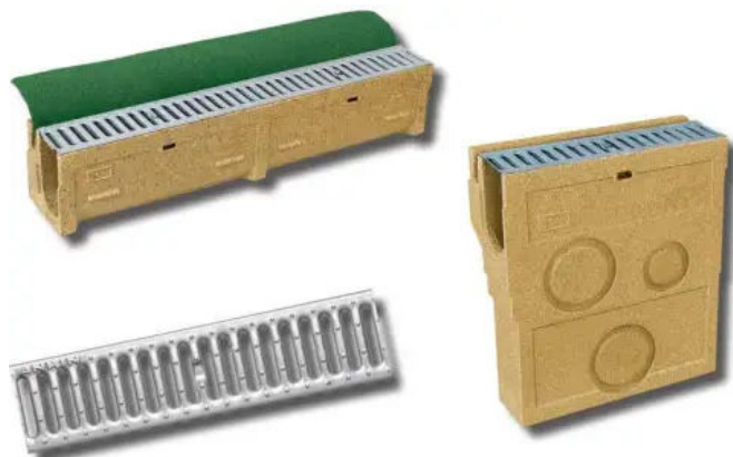
NW 100 für rechteckige Kunstrasenspielfelder
