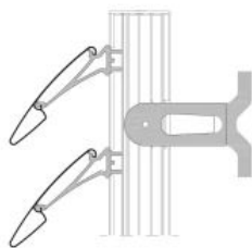
WICSOLAIRE - Lamellen mit Tragkonstruktion (©WICONA)
