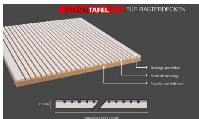
Aufbau: StudioLine Plus Systemtafeln
