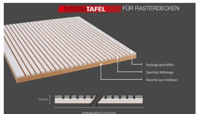
Aufbau: StudioLine Plus Systemtafeln
