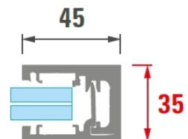
Systemschnitt
