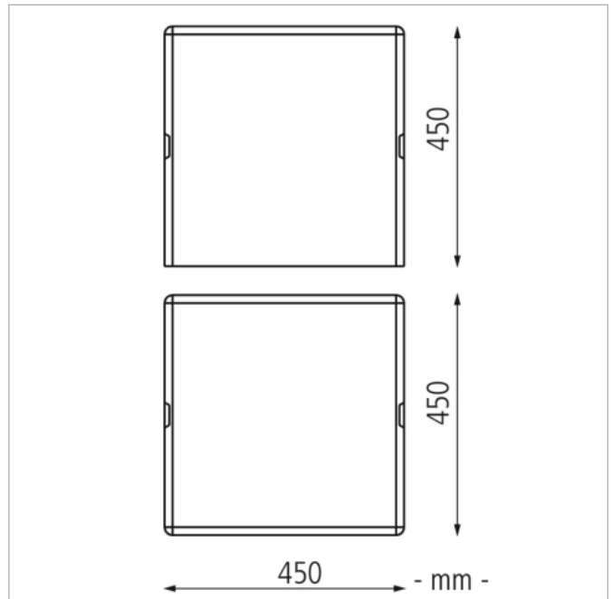
Sitzpoller IDRA - Maßskizze
