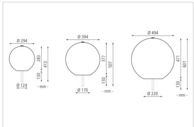
Poller SFERA - Maßskizze
