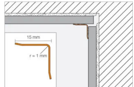
Schlüter®-ECK-KI für Innenecken
