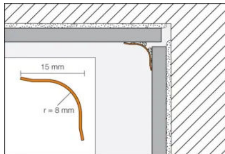
Schlüter®-ECK-KHK – als Hohlkehle ausgeprägtes Edelstahl-Eckprofil zum nachträglichen Aufkleben an Innenecken
