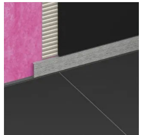
alferline Duschwandblende
