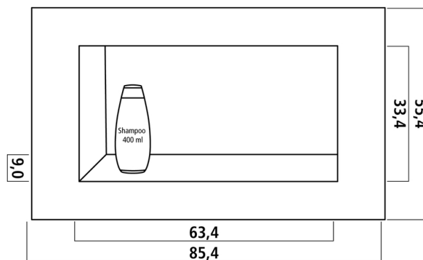
Sopro Board 3D L (Innenmaße: 33,4 × 63,4 × 9 cm; Außenmaße: 55,4 × 85,4 × 10 cm; Dicke Rahmenflansch: 10 mm)
