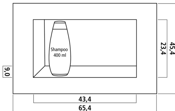
Sopro Board 3D S (Innenmaße: 23,4 × 43,4 × 9 cm; Außenmaße: 45,4 × 65,4 × 10 cm; Dicke Rahmenflansch: 10 mm)
