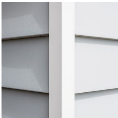
Hardie® NT3® Trim Faserzement-Profil für Außenecken Abmessungen: 3.655 × 90/140 × 25 mm
