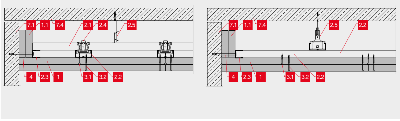
Wandanschluss - Querschnittschnitt Wandanschluss - Längsschnitt
