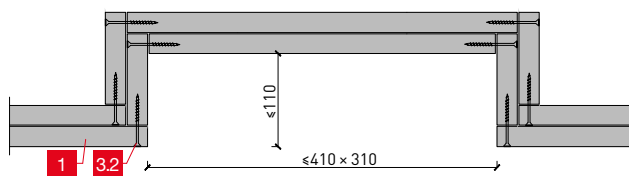
Lampenkasten
