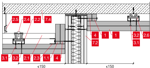
Anschluss an Trockenbauwand
