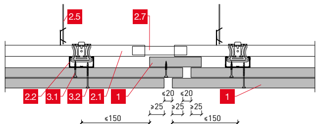
Bewegungsfuge
