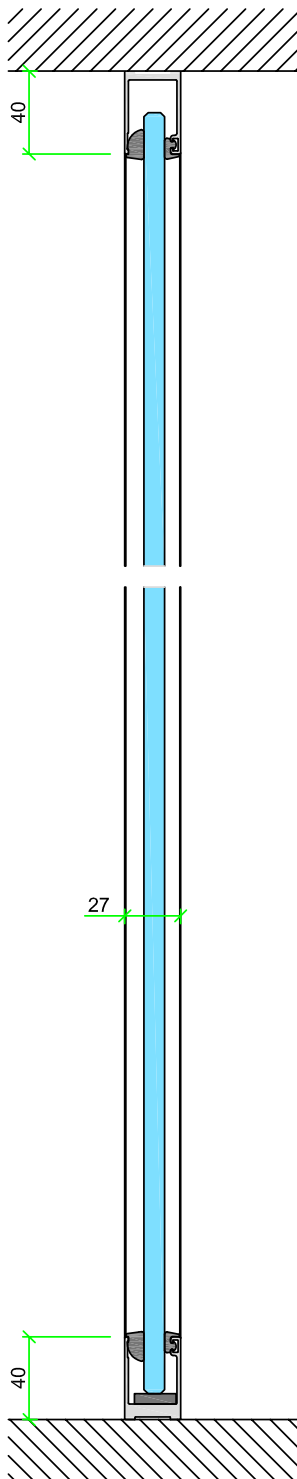
Vertikalschnitt T50
