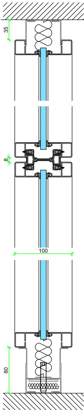
Vertikalschnitt T42
