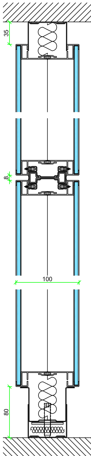
Vertikalschnitt T35
