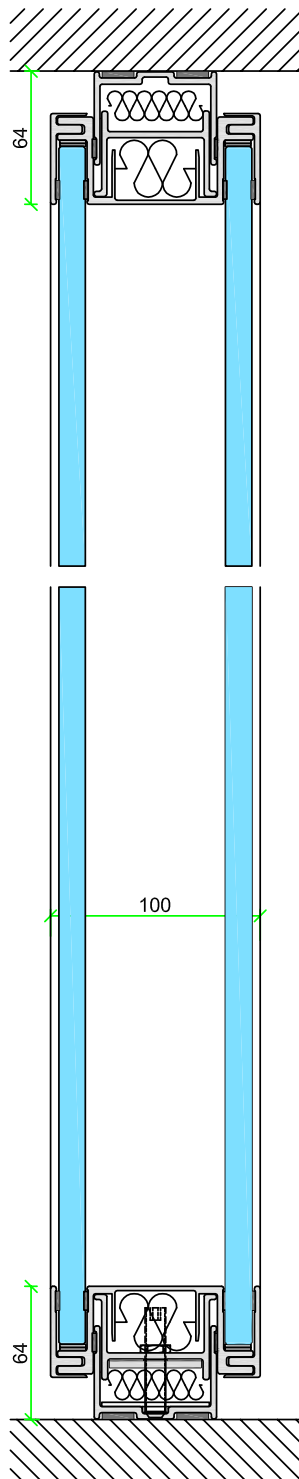
Vertikalschnitt T55
