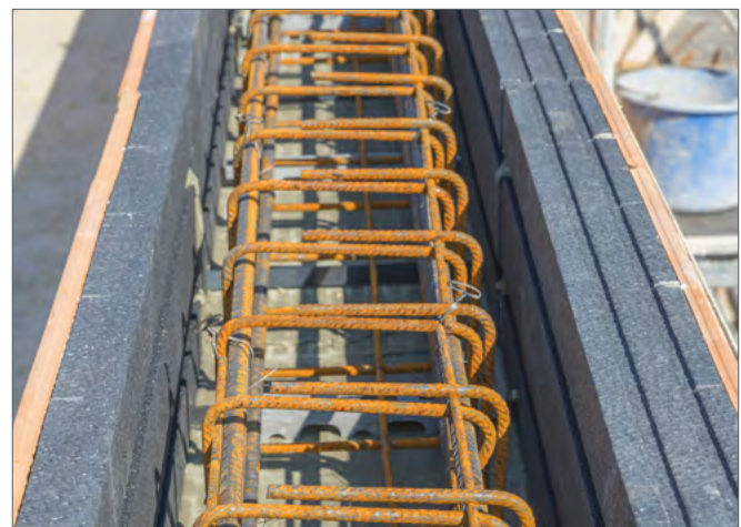
Abbildung 4.10: Zwei gedämmte Deckenrandschalen als Schalung für Ringbalken auf der Giebelwand
