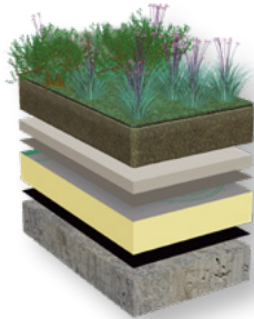
Dämmung unter Gründach
