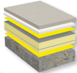
Wärmedämmung unter Estrich oder Fußbodenheizung
