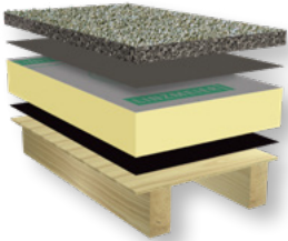
Dämmung unter Kies oder Terrassendach
