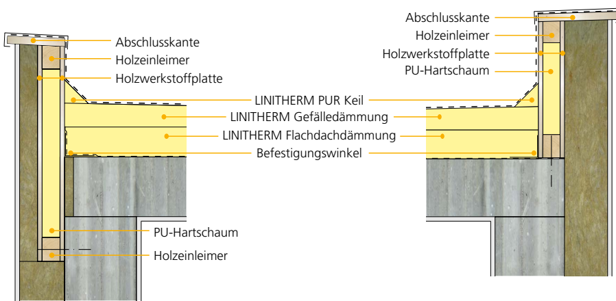
Attika-Element vorgehängt:
