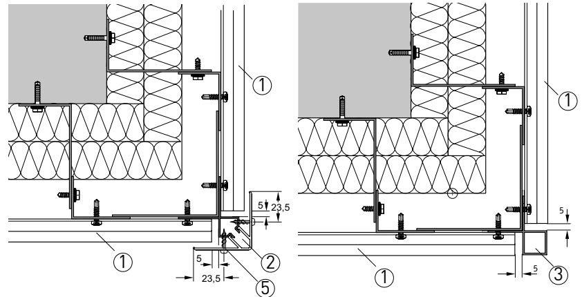
(A) Außenecke C, zweiteilig
