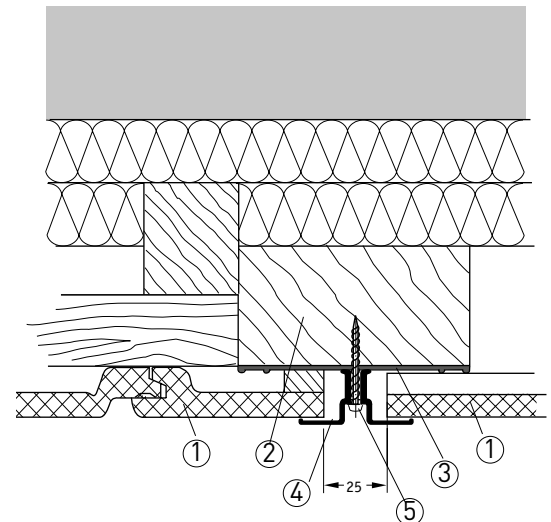
Ⓕ Senkrechter durchlaufender Stoß
