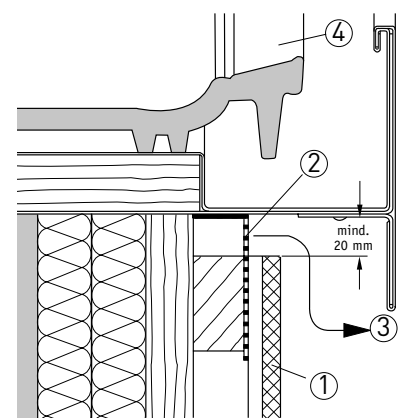
Ⓑ Anschluss an Giebedach
