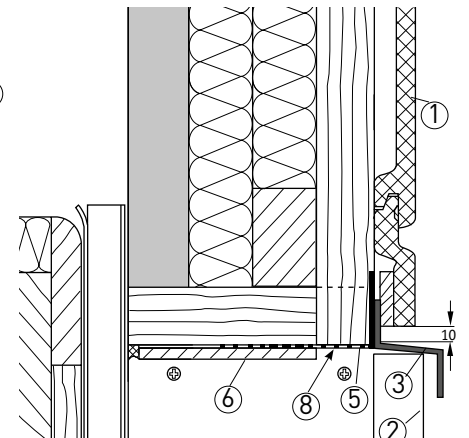
① Anschluss an Giebeldach
