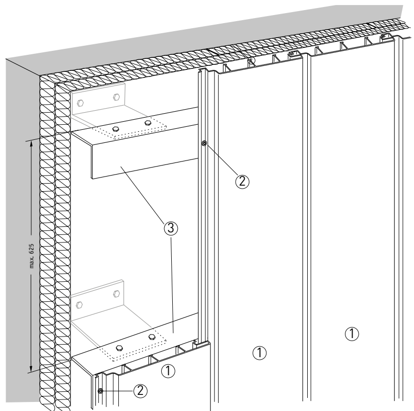
(D) Unterkonstruktion senkrechte Verlegung
