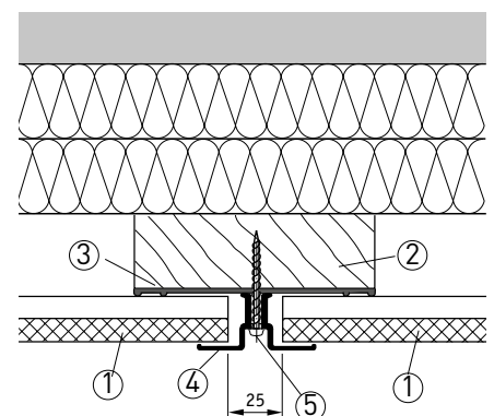
Ⓔ Abdeckprofil N + F
