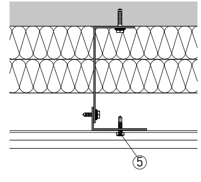
(B) Verschraubung an Alu-Unterkonstruktion
