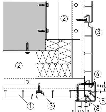
Ⓐ Außenecke C, zweiteilig
