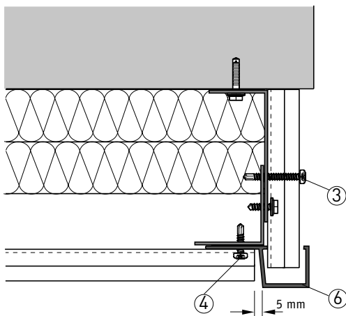
(E) Anschluss Fenstersturz Alternative
