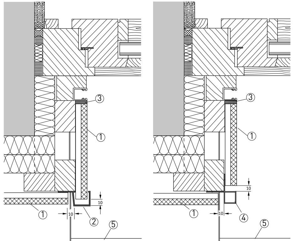
Ⓐ Anschluss Fensterlaibung
