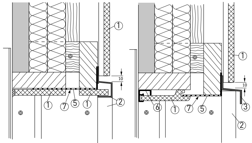
Ⓐ Anschluss Fenstersturz
