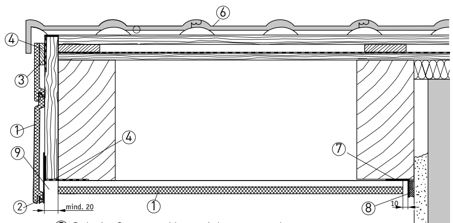
Ⓒ Schnitt Ortgang, Untersicht quer verlegt
