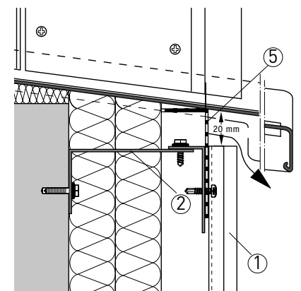
Ⓕ Anschluss Fensterbrüstung
