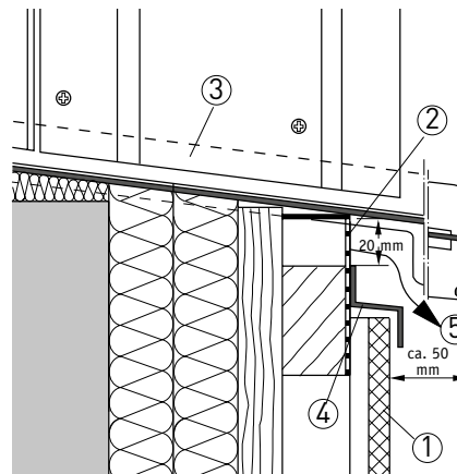
Ⓒ Anschluss Fensterbrüstung
