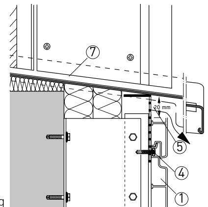
(D) Anschluss Fenstersturz
