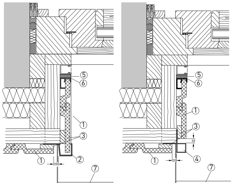
Ⓓ Anschluss Fenstersturz
