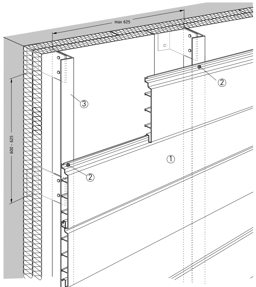
Ⓐ Unterkonstruktion waagrechte Verlegung
