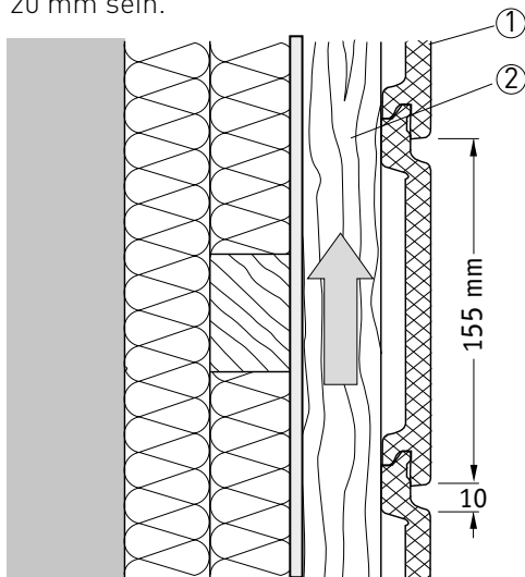
Ⓒ Unterkonstruktion
