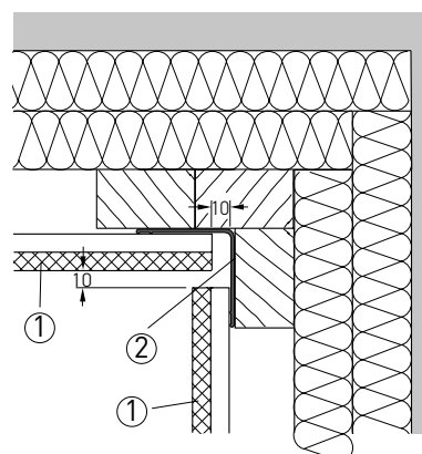
Ⓔ Innenecke
