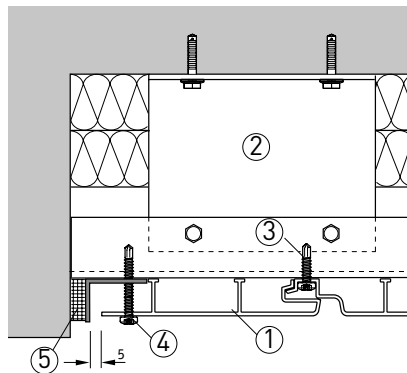
Ⓓ Anschluss seitlich in Nische
