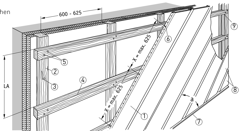
Ⓖ Verlegung diagonal
