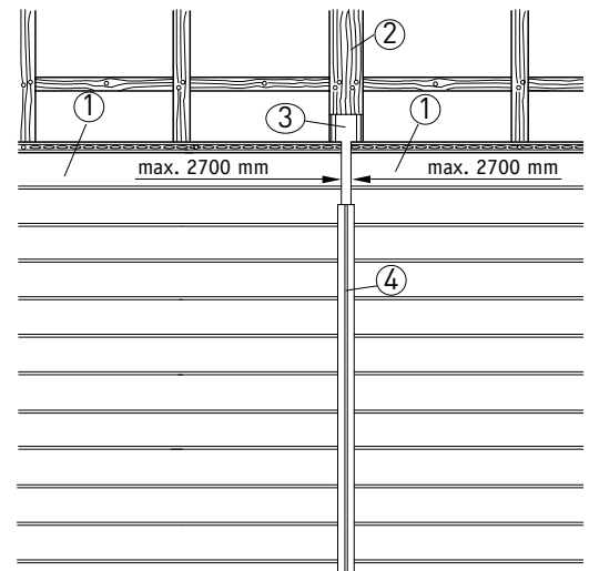
Ⓒ Ausklinkung der Nutwange
