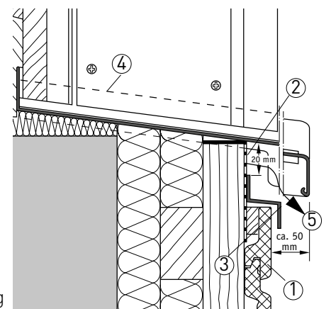
① Anschluss Fensterbrüstung
