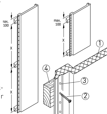
Ⓓ Befestigungsabstände
