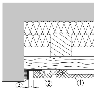
Ⓖ Anschluss an der Seite in der Nische
