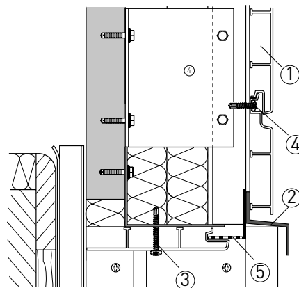
(D) Anschluss Fenstersturz
