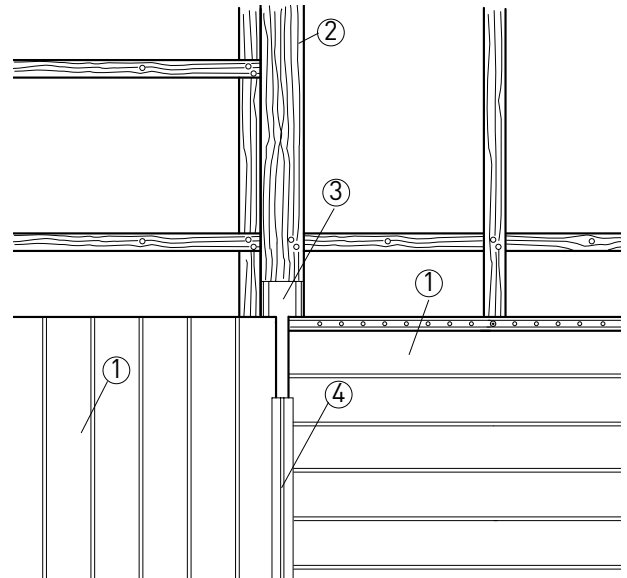
Ⓔ Senkrechte/waagerechte Verlegung
