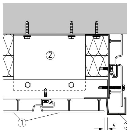
Ⓔ Anschluss Fenstersturz Alternative
