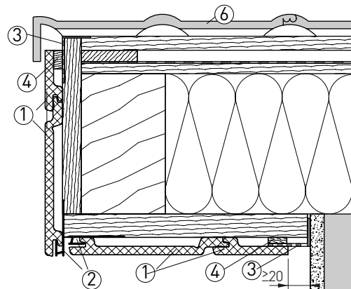
Ⓐ Schnitt Ortgang, Untersicht längs verlegt
