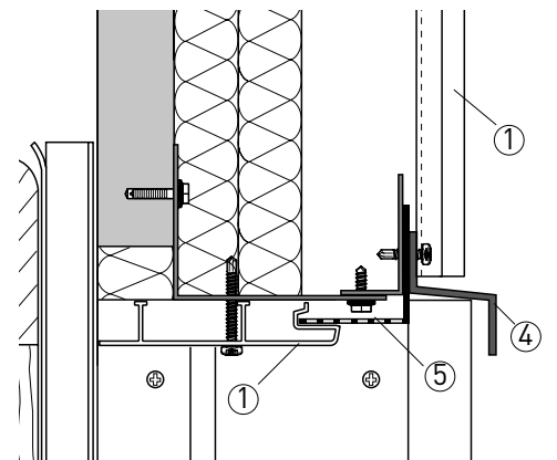
Ⓓ Anschluss Fenstersturz
