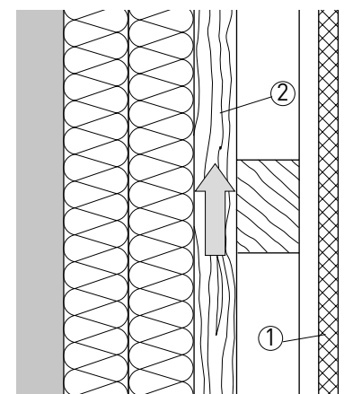
Ⓒ Senkrechter Schnitt
