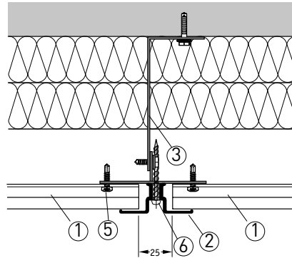
(A) Senkrecht durchlaufender Profilstoß
