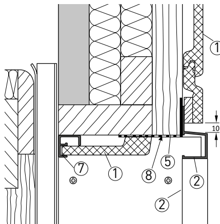
① Seitlicher Abschluss
