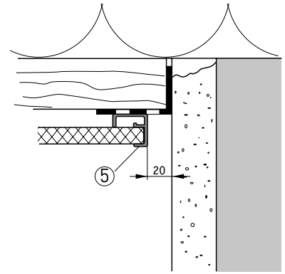
Ⓑ Wandanschluss Alternative
