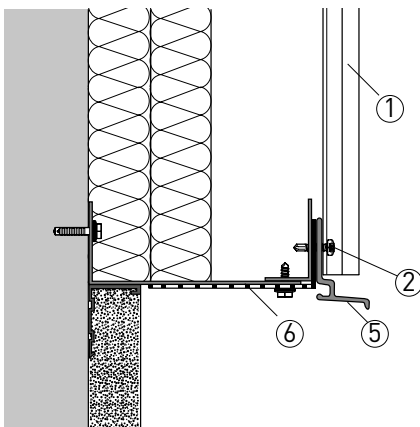
(E) Montagebeginn
