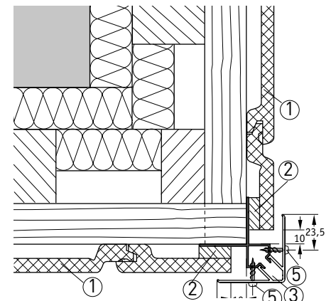
Ⓕ Außenecke, Alternative
