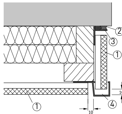
① Seitlicher Abschluss
