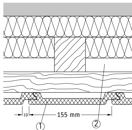
Ⓑ Waagerechter Schnitt
