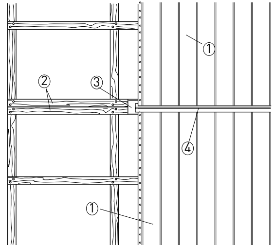
Ⓐ Senkrechte Verlegung
