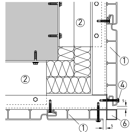
Ⓑ Außenecke, Alternative
