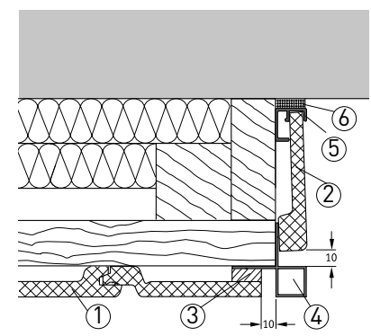
Ⓗ Seitlicher Abschluss
