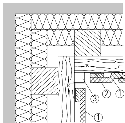
Ⓒ Innenecke
