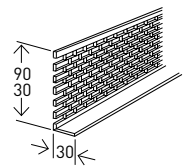
Lüftungsprofil
