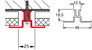
Abdeckprofil
