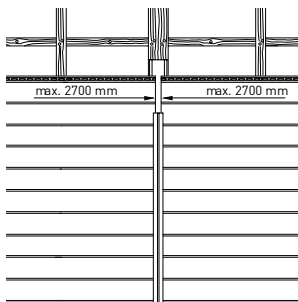
4. Horizontale Verlegung mit vertikaler Fuge, mit Abdeckprofil verkleidet
