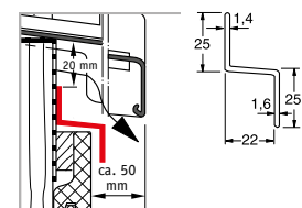
Z-Profil 2
