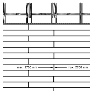
5. Horizontale Verlegung im Schiffsverband
