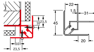
Außenecke C
