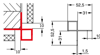
Alu-Außeneckprofil
