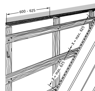
3. Diagonale Verlegung
