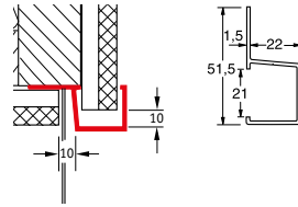
Anschlussprofil F
