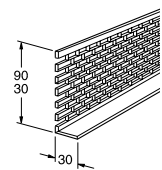
Lüftungsprofil
