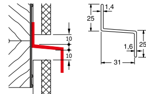
Z-Profil 1
