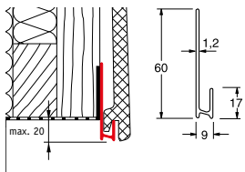
Anfangsprofil P
