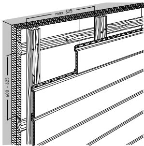
1. Horizontale Verlegung
