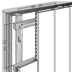
2. Vertikale Verlegung
