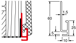
Anfangsprofil N + F
