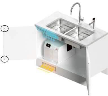
Falls der Sockel nicht min. 4 cm zurückgesetzt ist, muss ein zusätzliches Gitter für Abluft in die Sockelleiste eingesetzt werden
