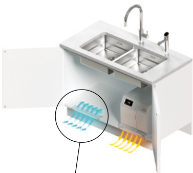
Optimal: Lüftungsgitter für Zuluft bei BCS 60 links vom Gerät, bei allen anderen Modellen rechts
