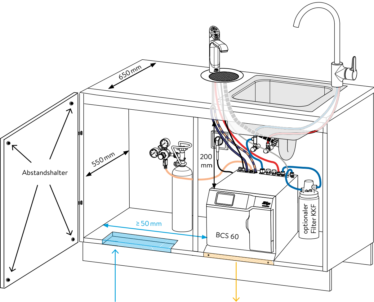
Ausschnitt am Schrankboden für Lüftungsgitter für Zuluft
