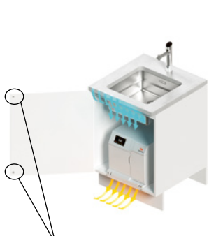
Bei geringer Nutzung reichen für die Zuluft Abstandhalter an der Tür (nicht bei BCS 60 und CS 100)
