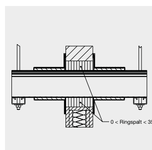
Kanal durchgängig Wandöffnung \geq Kanalquerschnitt
