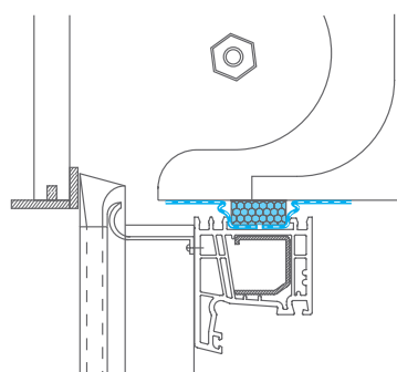
Fensteranschluss oben mit Rollladenkasten
