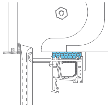
Fensteranschluss oben mit Rollladenkasten
