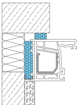
Mehrschalige Außenwand (Klinker)
