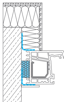
Wärmedämm- verbundsystem WDV
