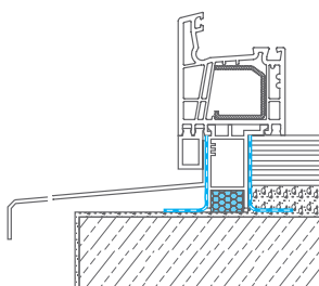
Fensteranschluss unten
