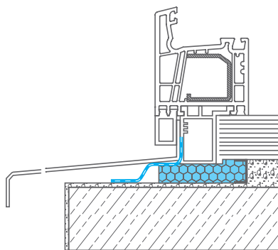
Fensteranschluss unten
