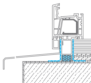
Fensteranschluss unten
