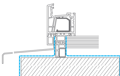
Fensteranschluss unten
