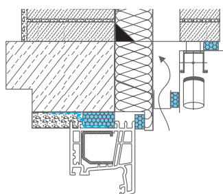
Fensteranschluss oben mit Jalousiekasten
