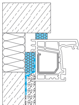
Mehrschalige Außenwand (Klinker)
