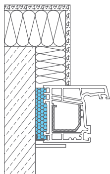
Wärmedämm- verbundsystem WDVS
