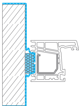
Einschaliges Mauerwerk
