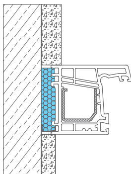
Einschaliges Mauerwerk
