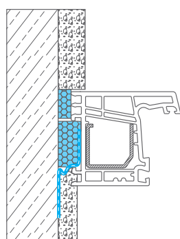
Einschaliges Mauerwerk
