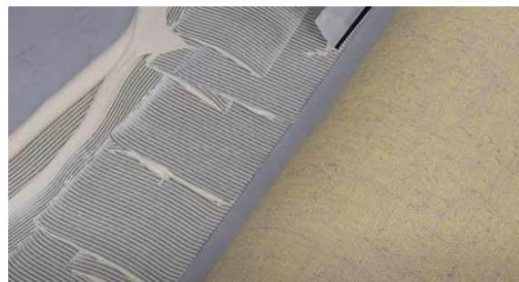
Klebstoffauftrag B1 Zahnung (TKB Ausführung, ca. 300 – 350 g/m 2 bei Belägen mit Juterücken)
