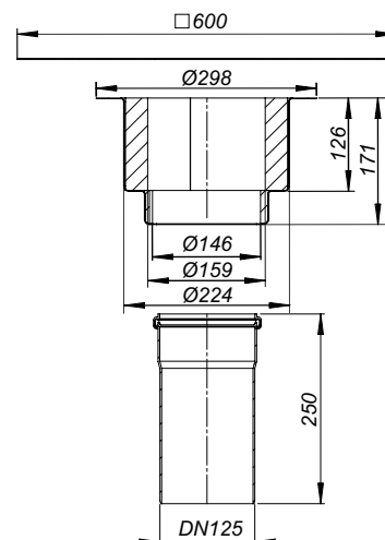
Brandschutzelement 10 Stahltrapez
