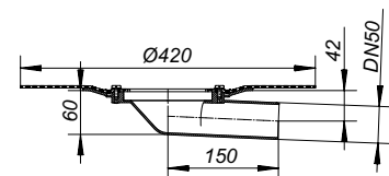
Balkonablaufgehäuse 83 DallBit
