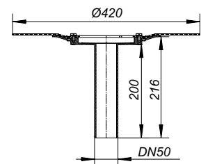
Balkonablaufgehäuse 84 DallBit
