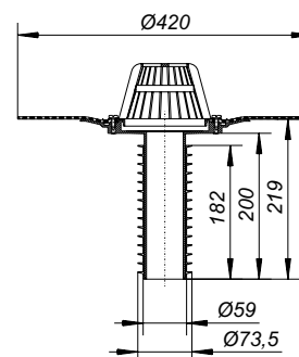
Sanierungs-Dachablauf 84 DallBit
