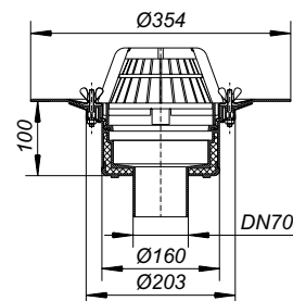
Aussparungsmaß: 265 x 320 mm Kernbohrungsmaß: Ø: 265 mm
