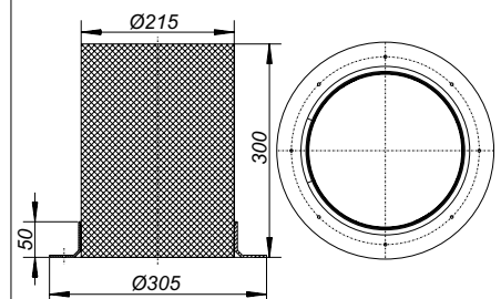
Deckendurchführung DD 200
