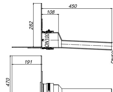
Attikaablauf DallBit DN 50
