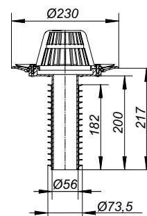
Sanierungs-Dachablauf 84 Schraubflansch
