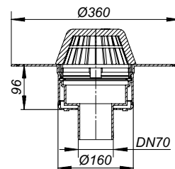
Dachablauf 62 PVC
