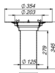
Aufstockelement 630 Schraubflansch
