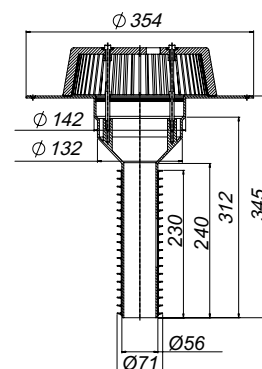
Sanierungs-Dachablauf 63 T FPO-PP
