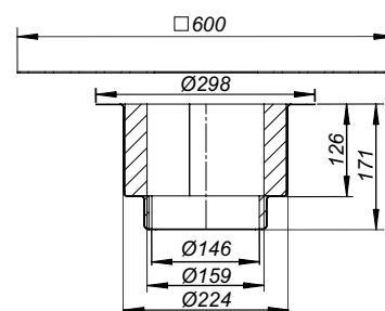
Brandschutzelement 9 Stahltrapez
