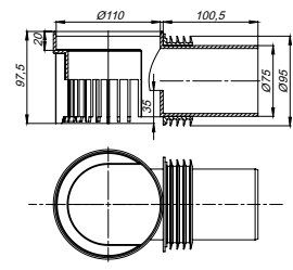
Notentwässerungselement für Attikaabläufe
