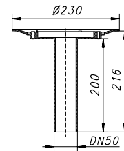
Balkonablaufgehäuse 84
