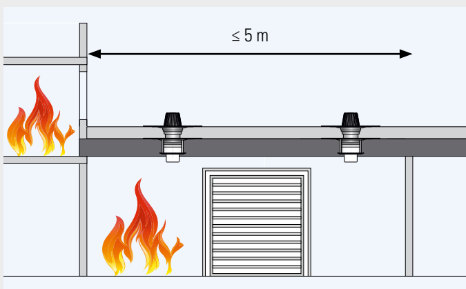
Bei Decken mit Anforderungen an eine Feuerwiderstandsdauer (F 30/60/90/120)
