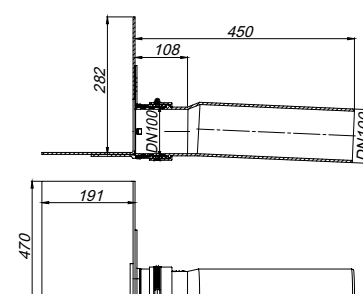
Attikaablauf DallBit DN 100
