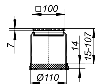
Aufsatz EC 10
