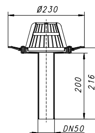
Dachablauf 84 D Schraubflansch
