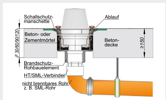
Brandschutz mit Dachablauf mit abZ Z-19.17-1800 und aBG Z-19.53-2602
