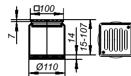
Aufsatz ECS 10
