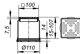
Aufsatz E 10
