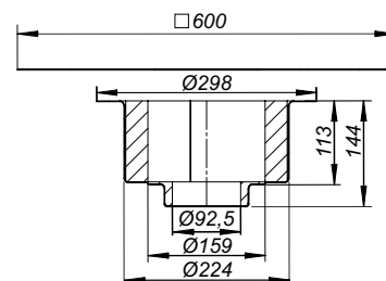
Brandschutzelement 8 Stahltrapez
