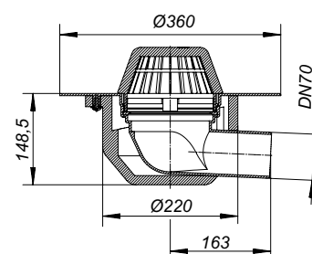
Dachablauf 64 FPO-PP
