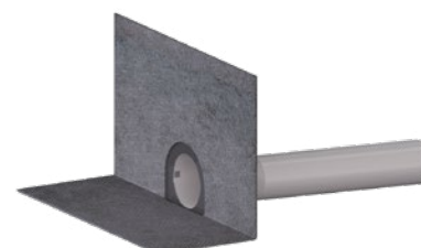
Attikaablauf DallBit DN 50
