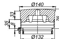
Notentwässerungseinheit 83/84
