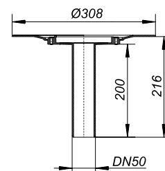
Balkonablaufgehäuse 84 FPO-PP
