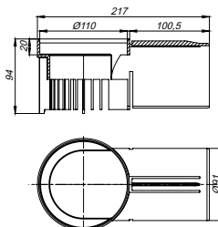
Entwässerungselement für Attikaabläufe
