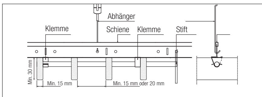
Deckenmontage
