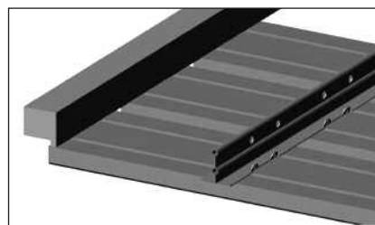
Decke mit Randanschluß
