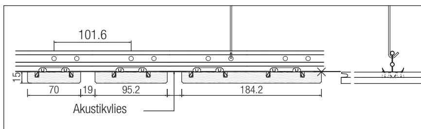
Deckenmontage
