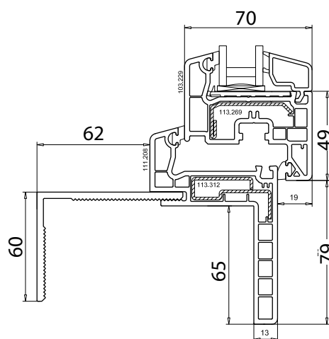
Typ Klickfix 70 TOP / MDK
