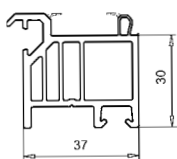
Fensterbankanschlussprofil 3 cm Neubau
