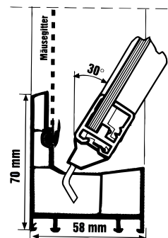
Profilquerschnitt Typ PLUS Flügel in Kippstellung
