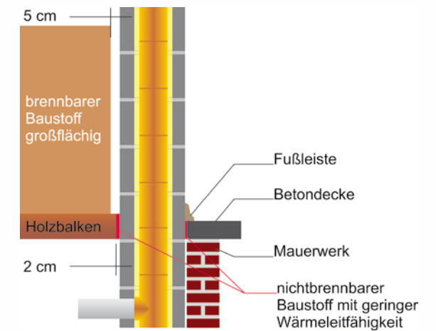
Beispiel für Abstände zu brennbaren Bauteilen bei der Schornstein-Abstandsklasse G50.
