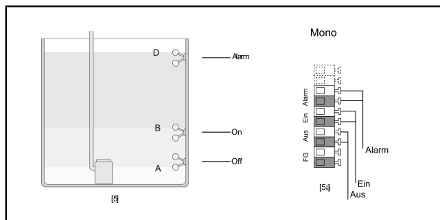
Afb. 1: Vlotterschakelaar Mono
