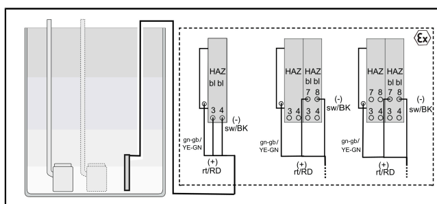
Fig. 8: Pegelsonde ATEX
