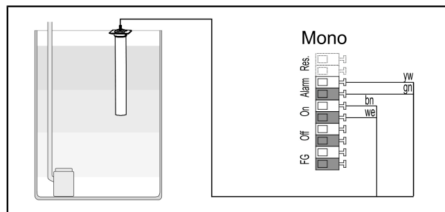
Abb. 4: Membrandruckschalter Mono
