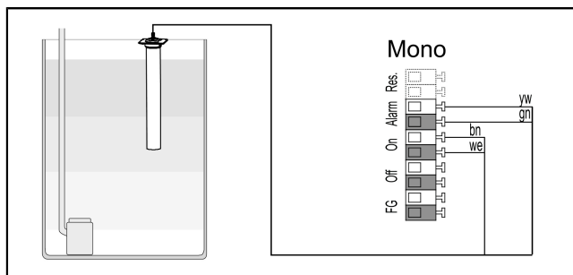
Afb. 4: Membraandrukschakelaar Mono
