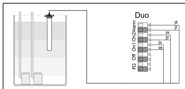
Fig. 5: Pressostato a membrana Duo
