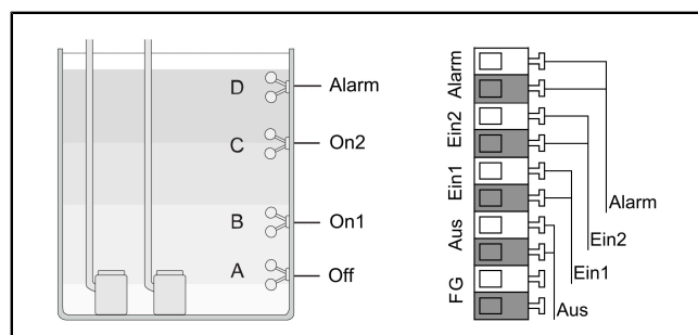
Rys. 2: Przełącznik pływakowy w urządzeniach typu Duo
