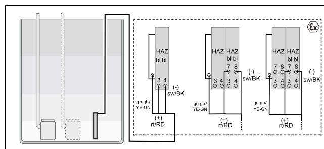
Afb. 8: Pegelsonde ATEX
