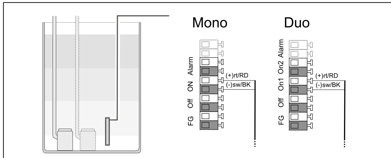
Afb. 3: Peilsonde aansluiten
