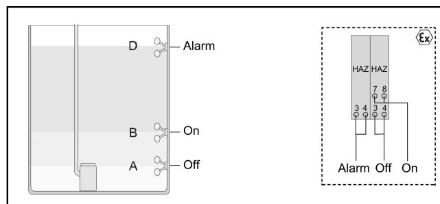
Rys. 6: Przełącznik pływakowy Mono ATEX
