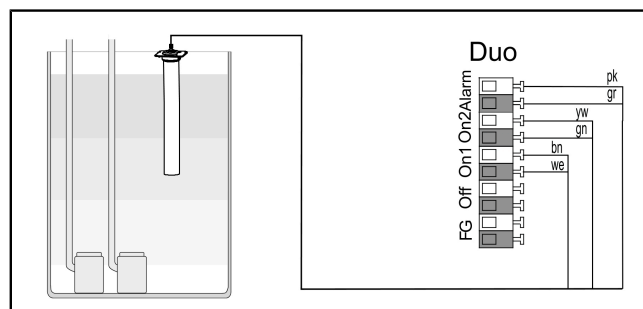
Abb. 5: Membrandruckschalter Duo
