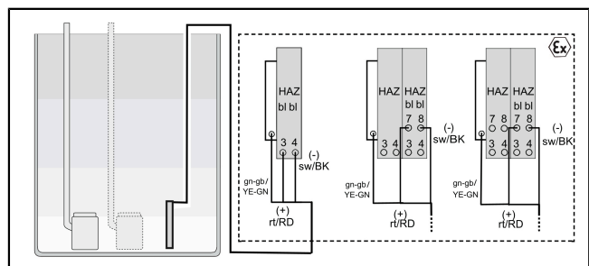
Abb. 8: Pegelsonde ATEX
