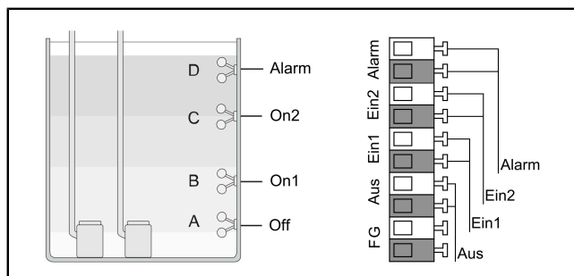
Afb. 2: Vlotterschakelaar Duo
