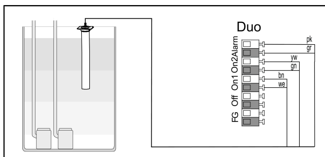
Afb. 5: Membraandrukschakelaar Duo
