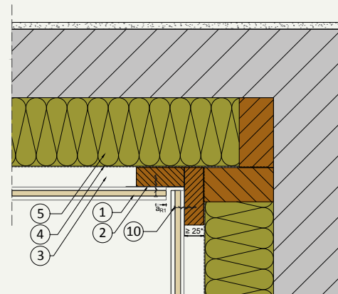
H.04 Innenecke
