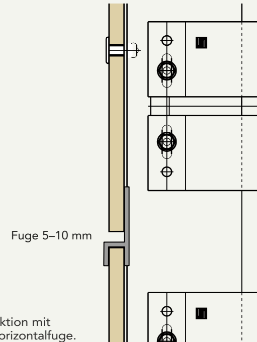
3. Metallunterkonstruktion, geschlossene Horizontalfuge.
