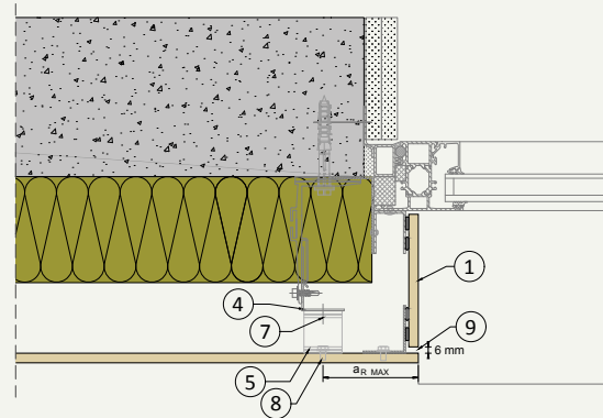
H.02 Laibungsanschluss
