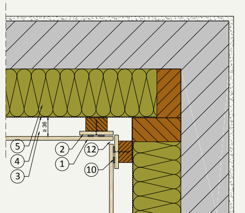
H.04 Innenecke
