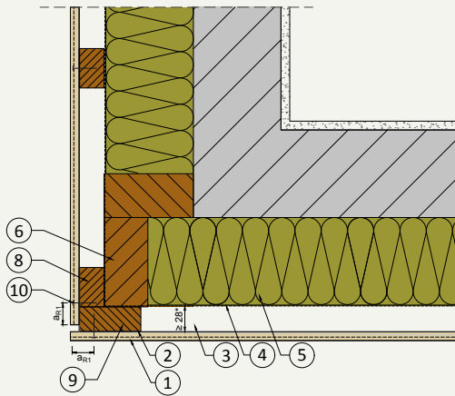
H.03 Außenecke
