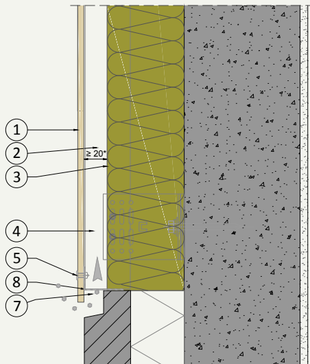
V.02 Sockelanschluss
