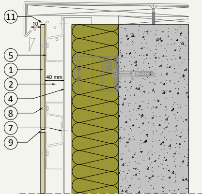
V.01 Dachanschluss (Attika)
