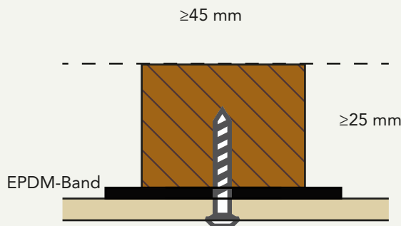
1. Befestigung auf Traglattung (min. 45x25 mm).
