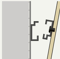
Verdeckte Befestigung
