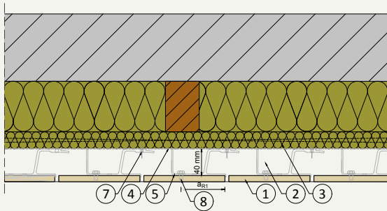
H.01 Schnitt durch vertikale Fuge
