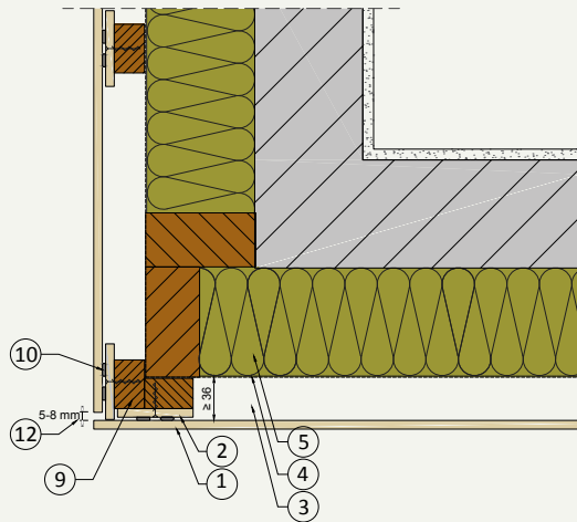
H.03 Außenecke
