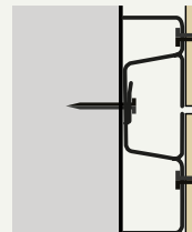
PlankClip auf Alu-UK
