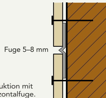
2. Holzunterkonstruktion mit halbgeschlossener Horizontalfuge.
