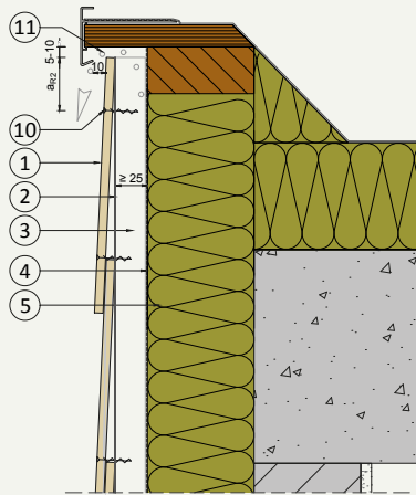
V.01 Dachanschluss (Attika)
