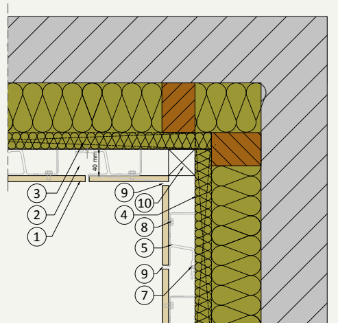
H.04 Innenecke
