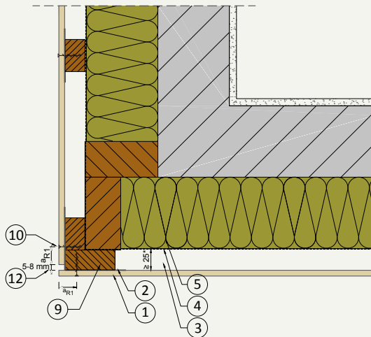
H.03 Außenecke
