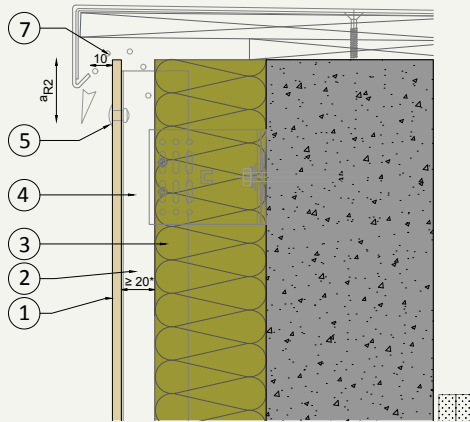
V.01 Dachanschluss (Attika)
