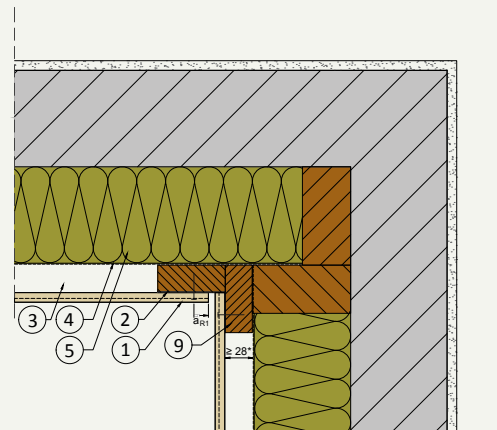
H.04 Innenecke
