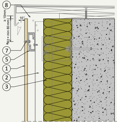
V.01 Dachanschluss (Attika)
