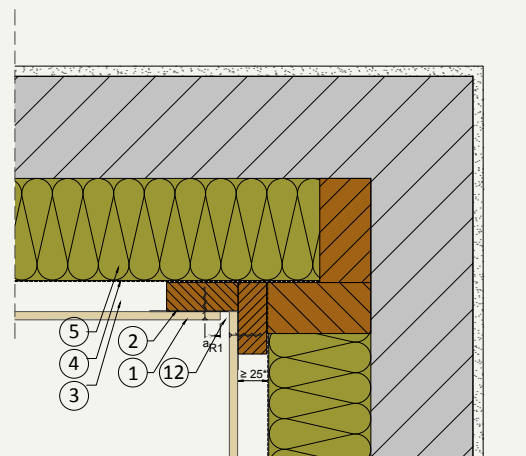
H.04 Innenecke
