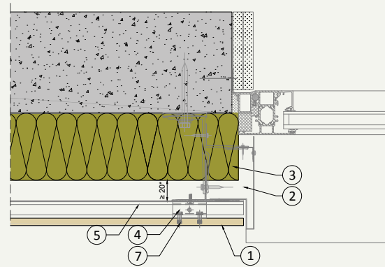
H.02 Laibungsanschluss
