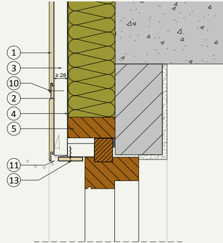
V.03 Oberer Fensteranschluss (Sturz)
