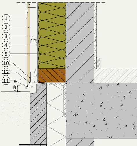
V.02 Sockelanschluss
