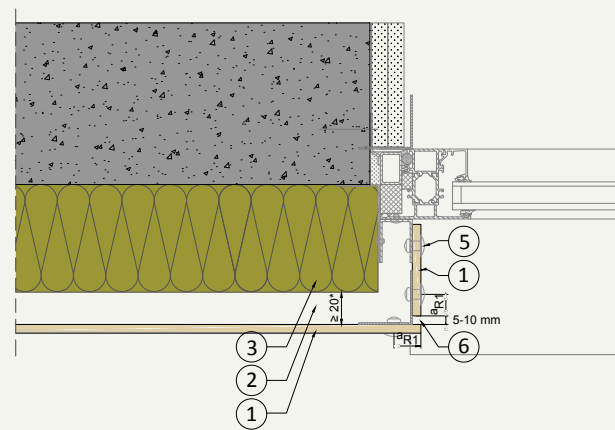
H.02 Laibungsanschluss
