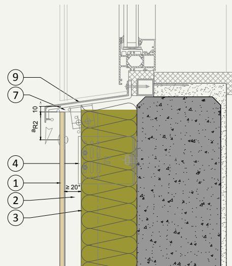
V.04 Unterer Fensteranschluss (Brüstung)
