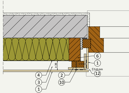
H.02 Laibungsanschluss
