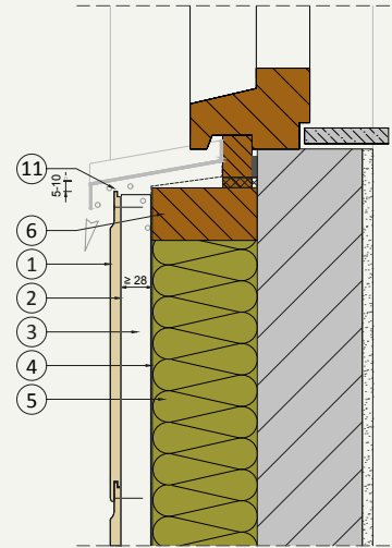
V.04 Unterer Fensteranschluss (Brüstung)
