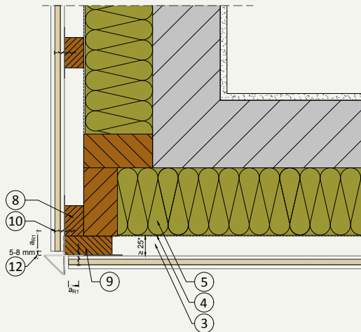
H.03 Außenecke
