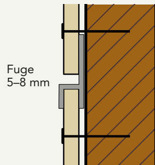
1. Holzunterkonstruktion mit geschlossener Horizontalfuge.
