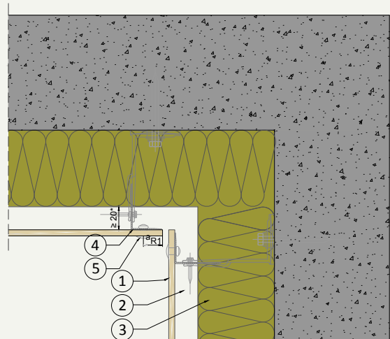
H.04 Innenecke
