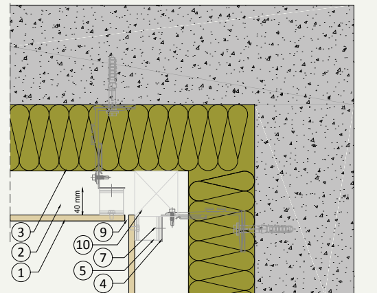
H.04 Innenecke
