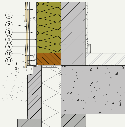
V.02 Sockelanschluss
