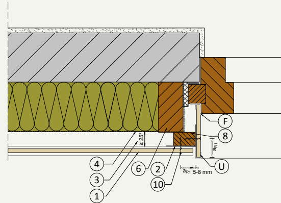
H.02 Laibungsanschluss
