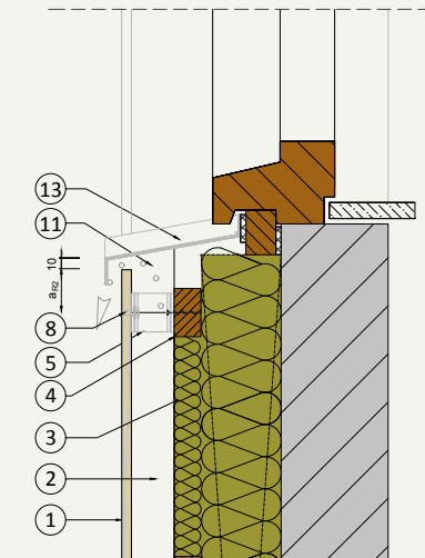
V.04 Unterer Fensteranschluss (Brüstung)
