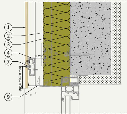
V.03 Oberer Fensteranschluss (Sturz)
