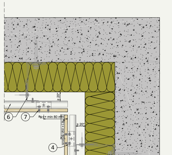
H.04 Innenecke
