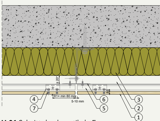
H.01 Schnitt durch vertikale Fuge
