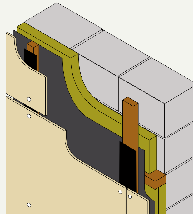
Unterkonstruktion aus Holz.
