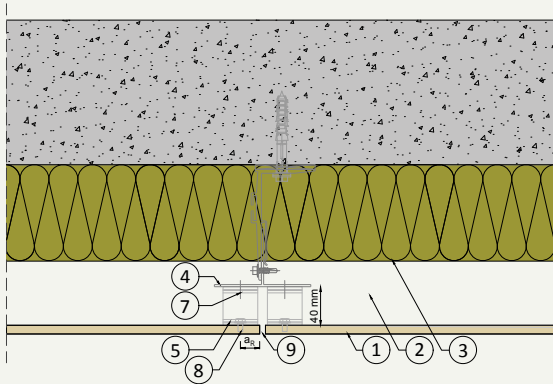
H.01 Schnitt durch vertikale Fuge
