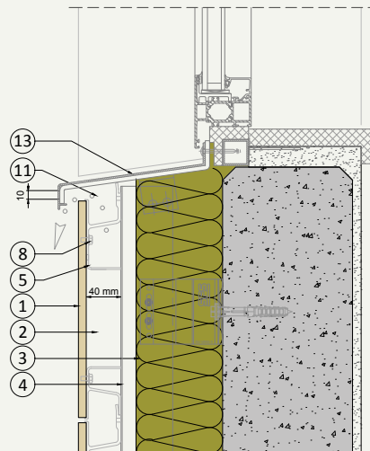
V.04 Unterer Fensteranschluss (Brüstung)
