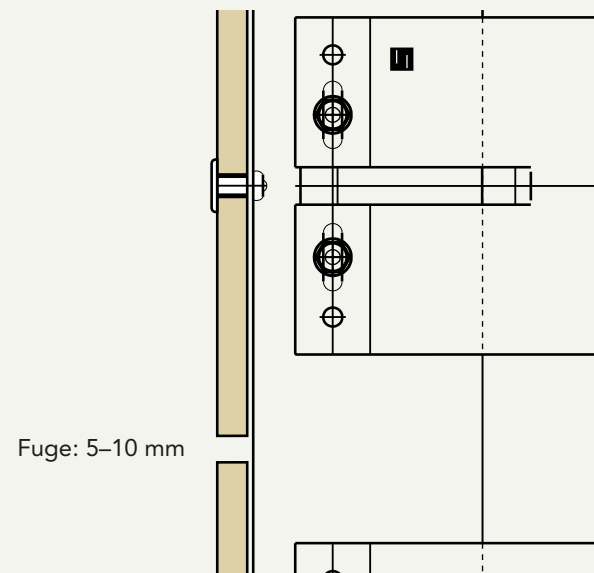
2. Metall-Unterkonstruktion, offene horizontale Fuge.
