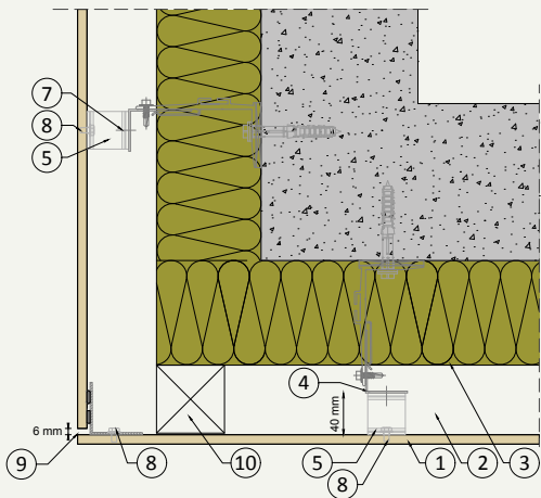
H.03 Außenecke
