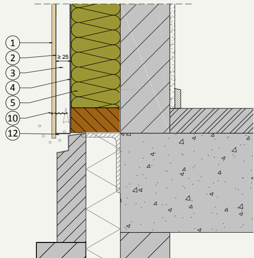
V.02 Sockelanschluss
