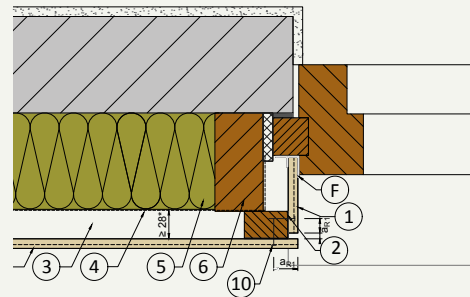
H.02 Laibungsanschluss
