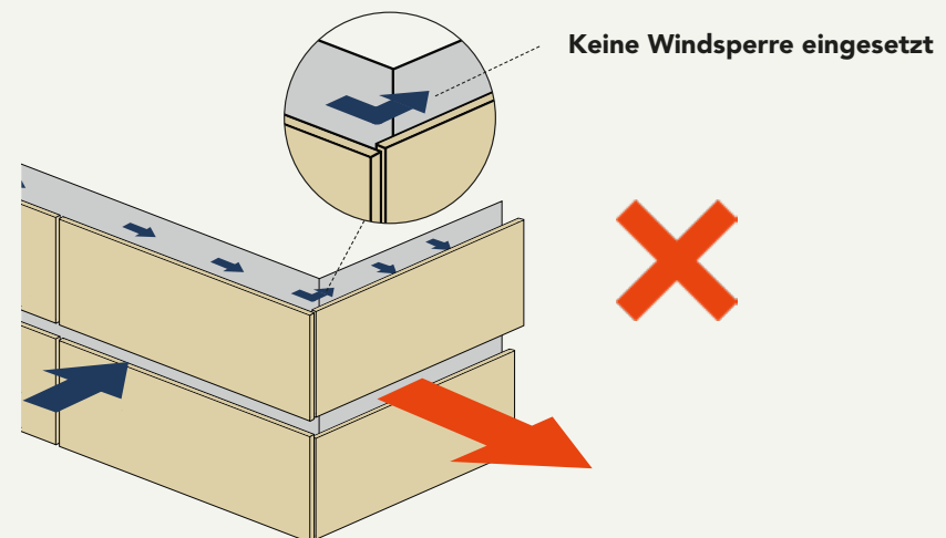
2. Fehlende Windsperre führt zu erhöhten Windlasten durch den Innendruck
