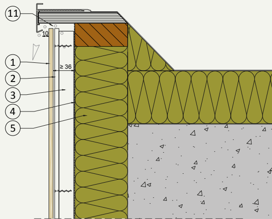
V.01 Dachanschluss (Attika)
