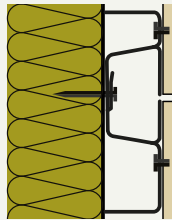
PlankClip auf Holz-UK
