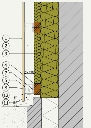
V.02 Sockelanschluss
