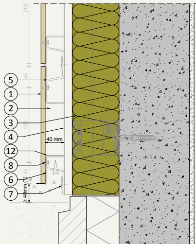
V.02 Sockelanschluss
