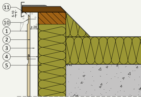
V.01 Dachanschluss (Attika)
