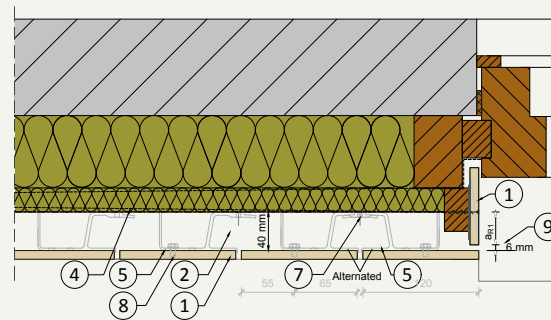
H.02 Laibungsanschluss
