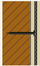
Klebesystem auf Holz-UK
