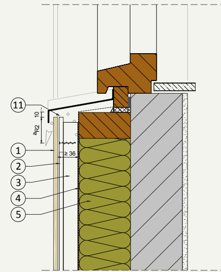
V.04 Unterer Fensteranschluss (Brüstung)
