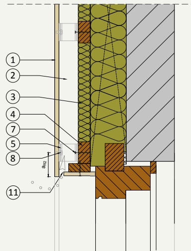
V.03 Oberer Fensteranschluss (Sturz)
