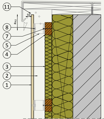
V.01 Dachanschluss (Attika)
