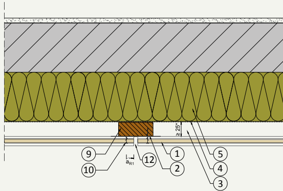
H.01 Schnitt durch vertikale Fuge
