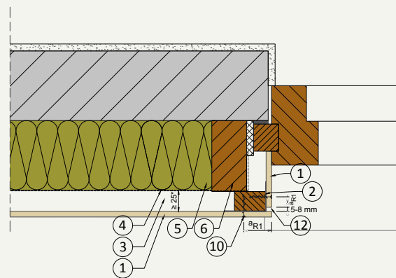
H.02 Laibungsanschluss
