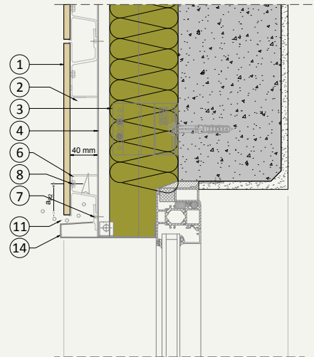
V.03 Oberer Fensteranschluss (Sturz)
