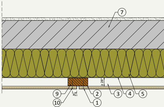
H.01 Schnitt durch vertikale Fuge
