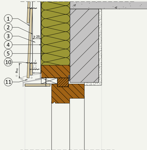
V.03 Oberer Fensteranschluss (Sturz)
