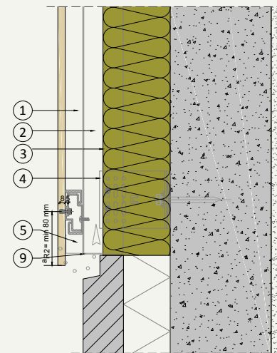
V.02 Sockelanschluss
