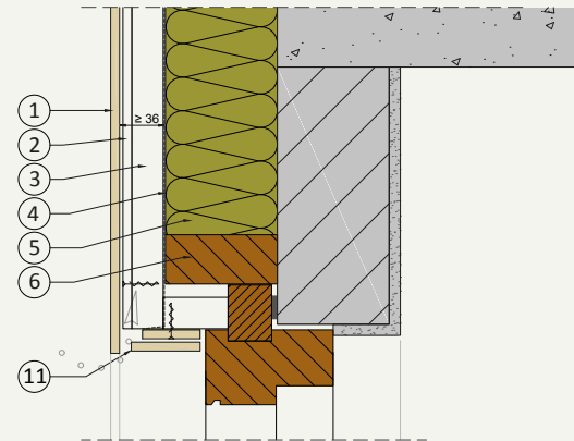
V.03 Oberer Fensteranschluss (Sturz)
