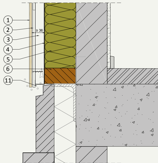
V.02 Sockelanschluss
