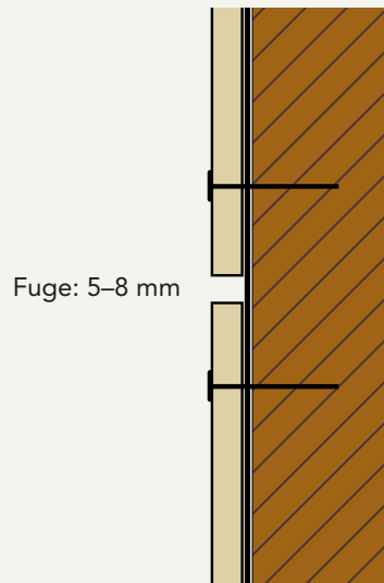
1. Unterkonstruktion aus Holz, offene horizontale Fuge.
