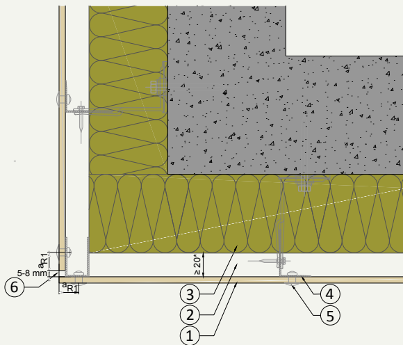
H.03 Außenecke
