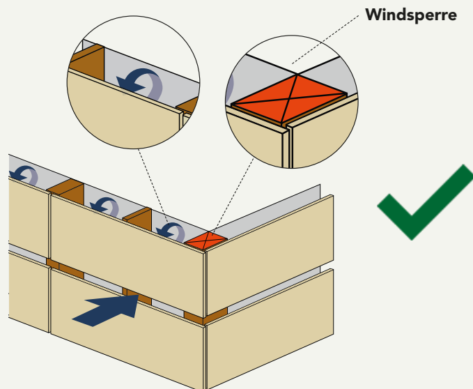
1. Windsperre korrekt angewendet
