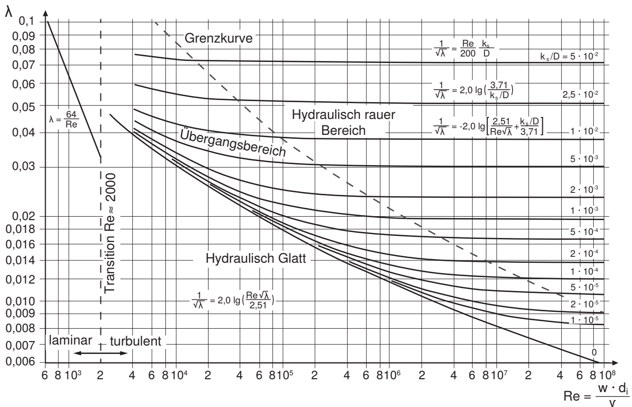
Abbildung 7: Moody-Diagramm
