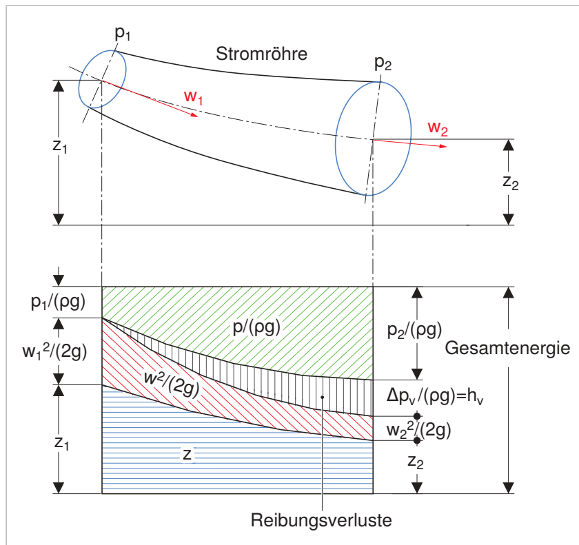
Abbildung 5: Graphische Darstellung der Bernoulli'schen Energiegleichung für reibungsfreie inkompressible Strömungen mit Verlustglied
