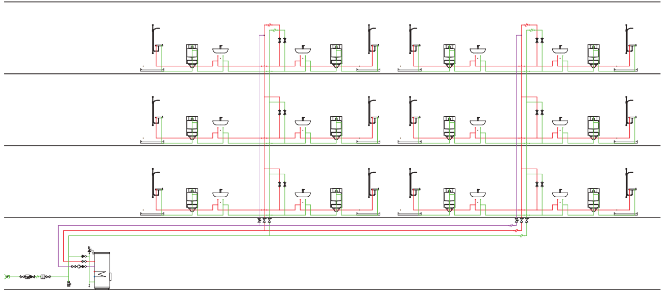
Abbildung 46: Vertikales Verteilkonzept mit seitlicher Einspeisung
