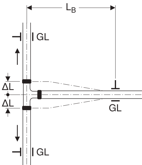
Abbildung 82: Dehnungsausgleich bei Abgangsleitung
