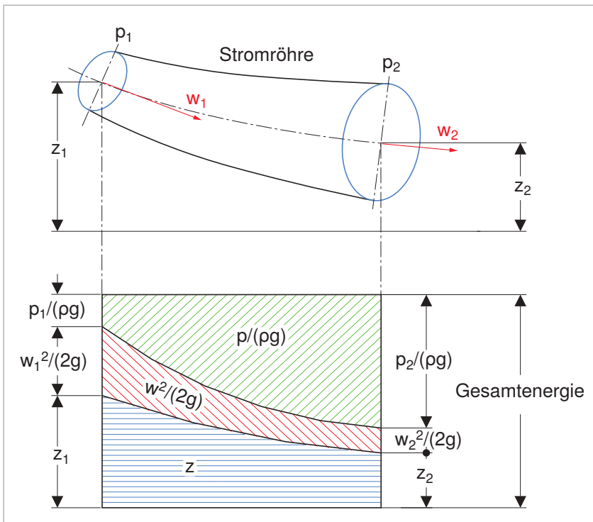
Abbildung 4: Graphische Darstellung der Bernoulli'schen Energiegleichung für reibungsfreie inkompressible Strömungen
