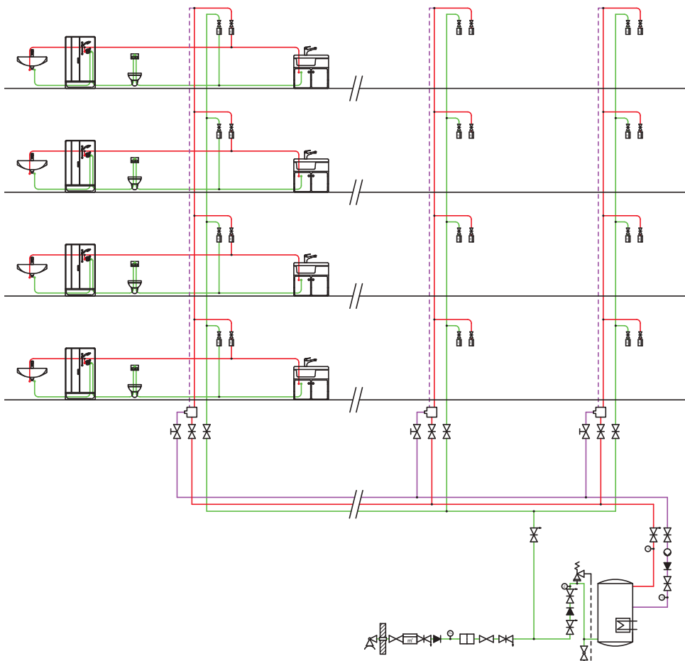
Abbildung 53: Innenliegende Zirkulation im Schacht
