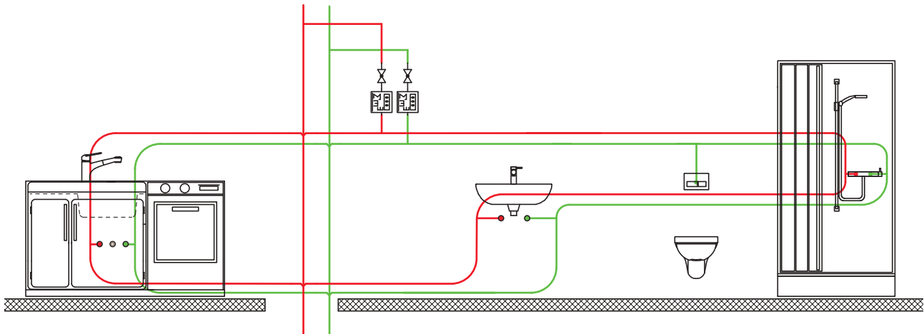
Abbildung 60: Stockwerksinstallation mit Ringleitung
