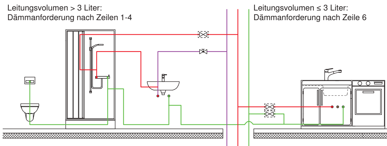
Abbildung 72: 3-Liter-Regel: Dämmung von zirkulierenden und nicht zirkulierten Stockwerksleitungen
