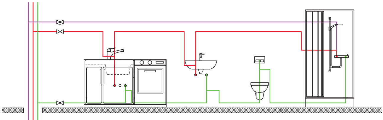
Abbildung 62: Thermisch entkoppelte Leitungsführung mit MasterFix Anschlüssen
