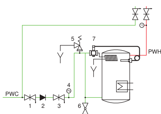
Indirekt beheizt
