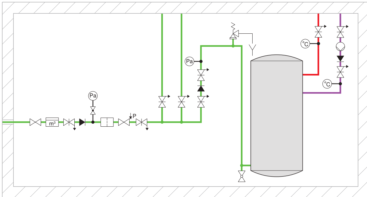
Abbildung 37: Beispiel Schema Hausanschlussraum / Technikraum
