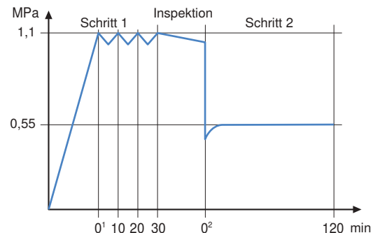
Abbildung 94: Druckprüfung von PP-, PE-, PE-X- und PB-Rohrleitungen sowie damit kombinierten Installationen aus Metall- und Mehrschichtverbund-Rohrleitungen
