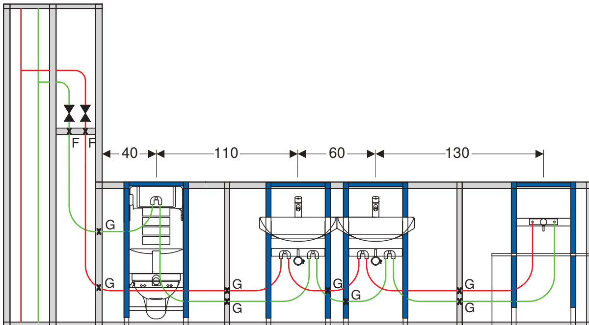
Abbildung 85: Befestigung von Systemrohren PB in Vorwandinstallationen
