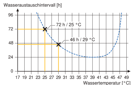
Abbildung 34: Wasseraustauschfunktion für Kaltwasserleitungen in Abhängigkeit der Temperatur
