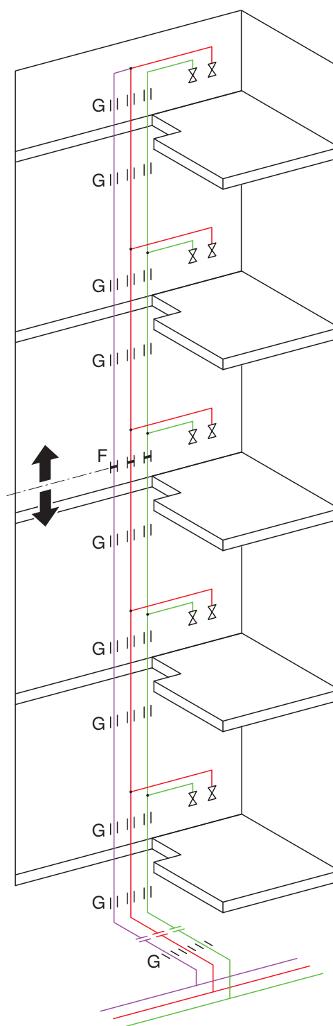
Abbildung 79: Steuerung der Längenausdehnung mit Fixpunkt im mittleren Stockwerk
