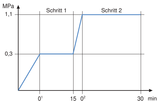
Abbildung 93: Druckprüfung von Metall- und Mehrschichtverbundrohren mit Pressverbindungen
