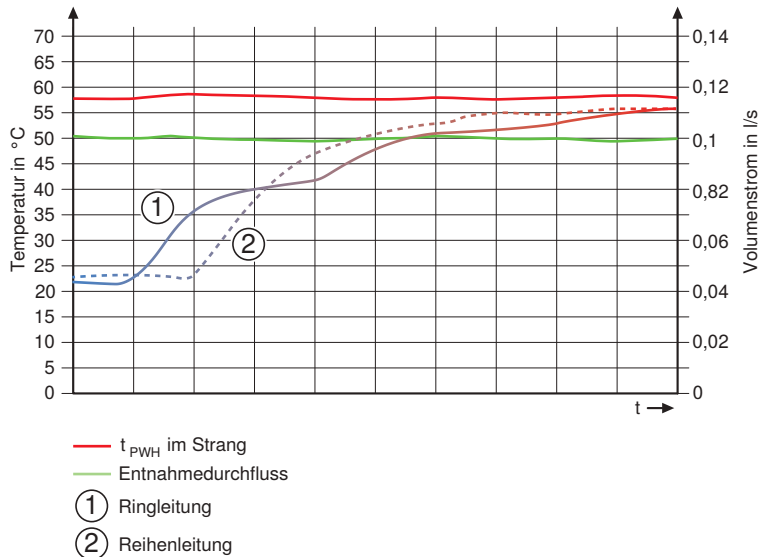
Abbildung 61: Temperaturverlauf und Ausstoßzeit bei Reihen- und Ringleitung
