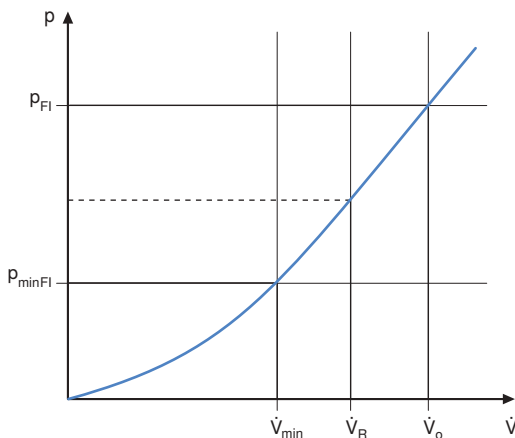
Abbildung 70: Mindestfließdruck und Berechnungsdurchfluss
