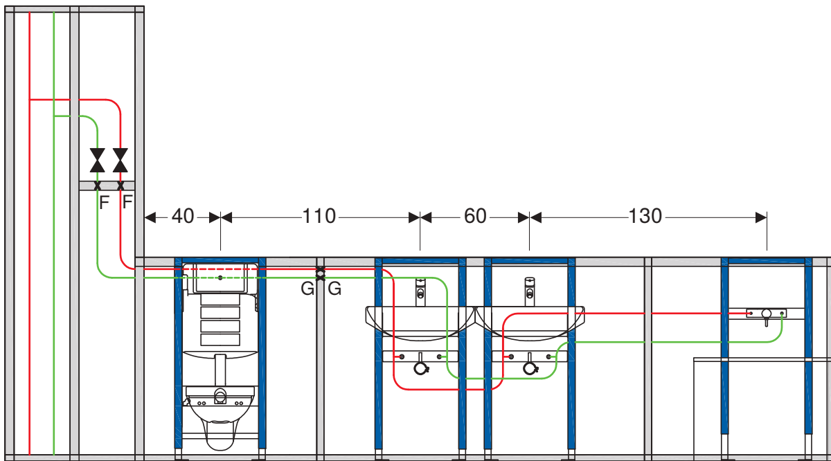
Abbildung 86: Befestigung von Systemrohren ML in Vorwandinstallationen
