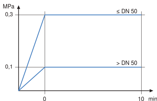
Abbildung 91: Belastungsprüfung mit ölfreier sauberer Druckluft oder Inertgas
