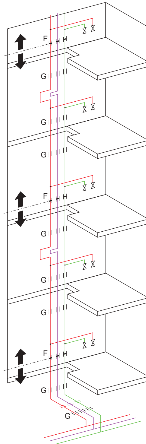
Abbildung 80: Steuerung der Längendeckung mit U-Rohrbogen und Unterteilung in Leitungsabschnitte
