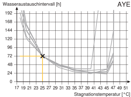
Abbildung 31: Auf 25 °C und 72 h standardisierte Wasseraustauschzeit in Abhängigkeit der Temperatur
