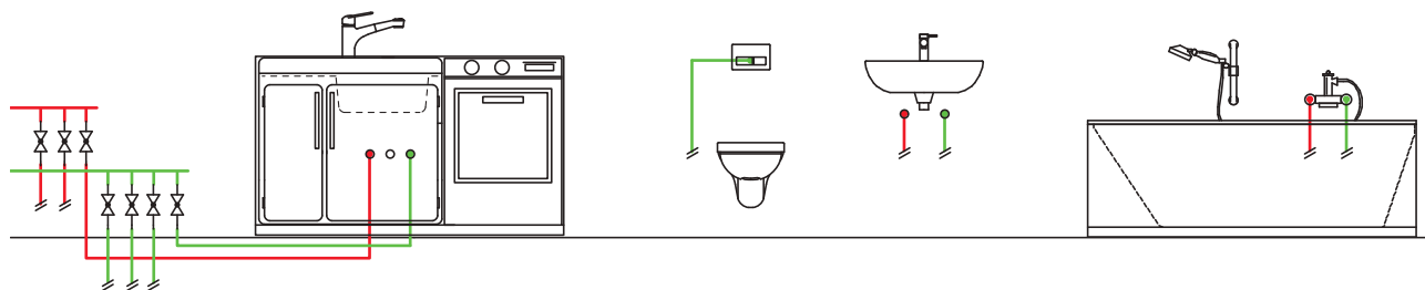
Abbildung 58: Stockwerksinstallation über Verteiler mit Einzelzuleitung
