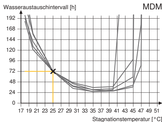
Abbildung 32: Auf 25 °C und 72 h standardisierte Wasseraustauschzeit in Abhängigkeit der Temperatur
