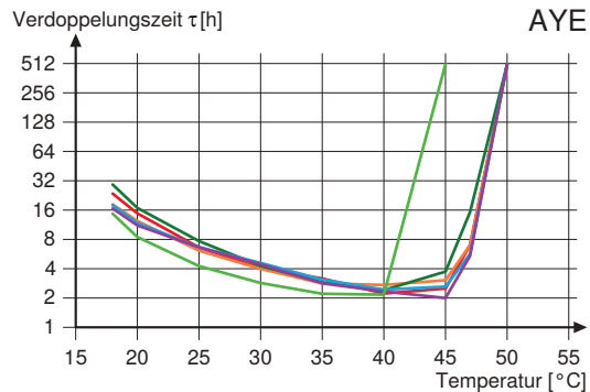
Abbildung 29: Logarithmische Darstellung der Verdoppelungszeit verschiedener Legionellenstämme in Abhängigkeit der Temperatur im Nährmedium AYE
