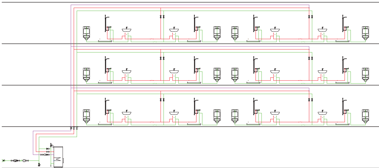
Abbildung 49: Horizontales Verteilkonzept
