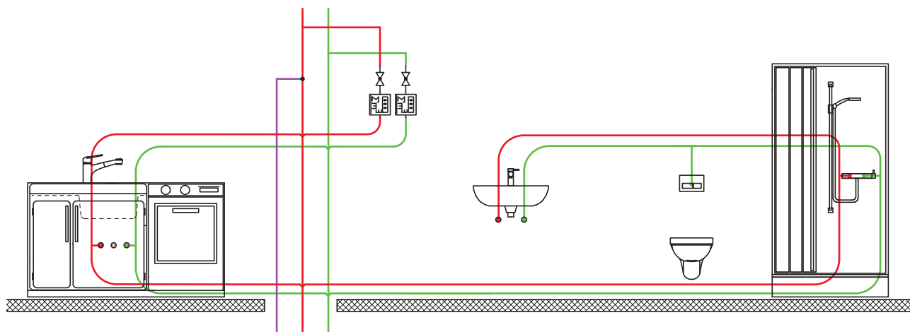
Abbildung 59: Stockwerksinstallation mit Reihenleitung
