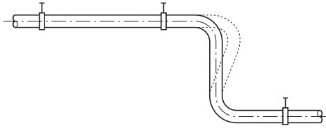
Abbildung 73: Aufnahme der Längenänderung \Delta L durch die Elastizität des Rohrleitungssystems
