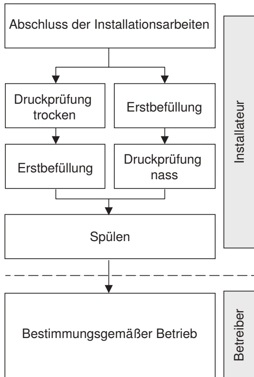
Abbildung 88: Teilaufgaben der Inbetriebnahme
