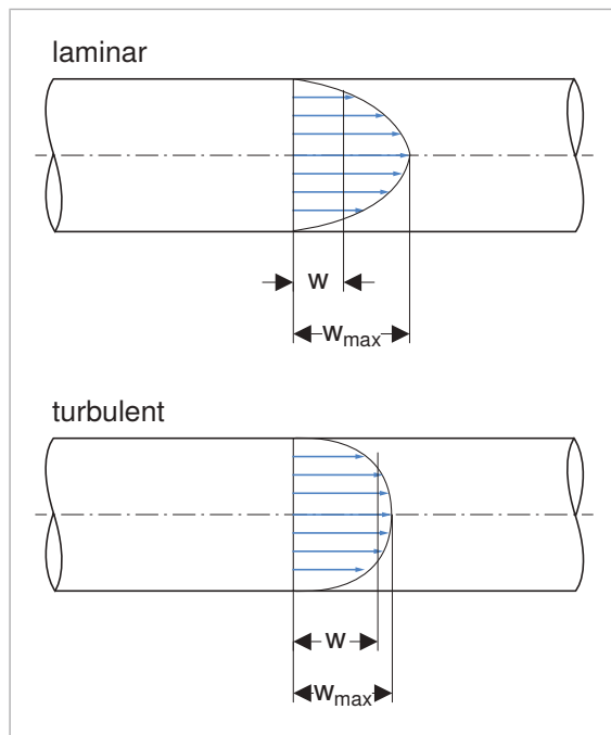
Abbildung 6: Geschwindigkeitsverteilung und mittlere Fließgeschwindigkeit w bei laminarer bzw. turbulenter Strömung
