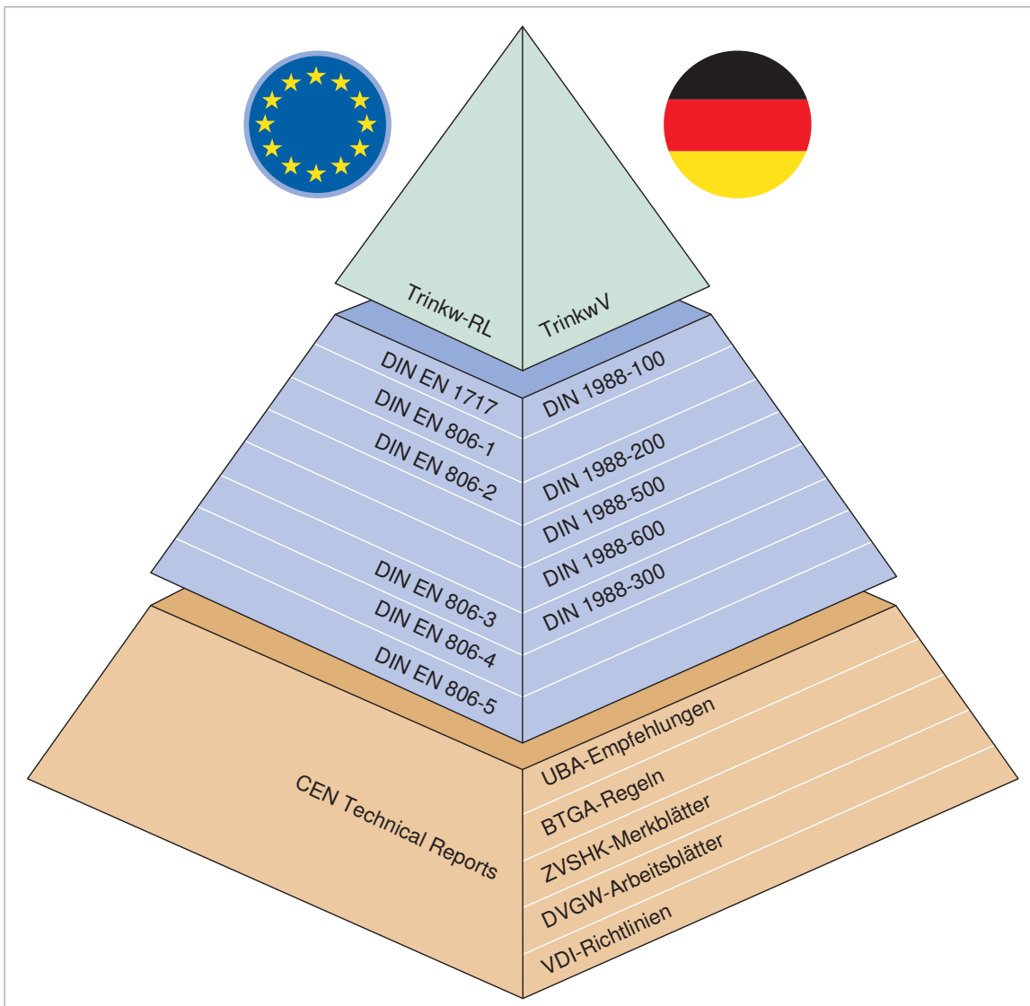
Abbildung 2: Zusammenspiel europäischer und nationaler Regelwerke
