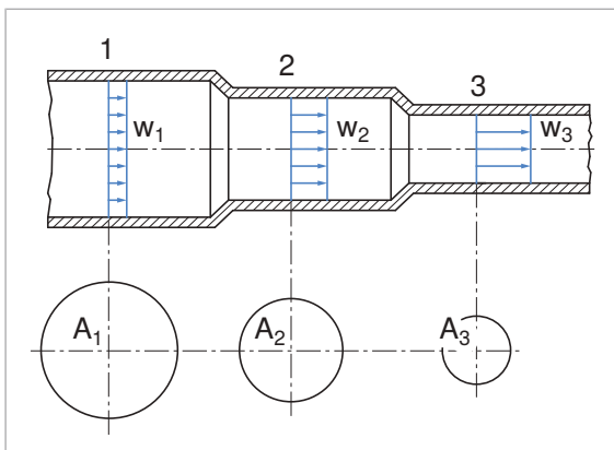
Abbildung 3: Graphische Darstellung der Kontinuitätsgleichung
