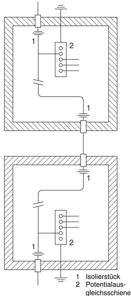
Abbildung 39: Potentialausgleich bei erdverlegten metallenen Rohrleitungen
