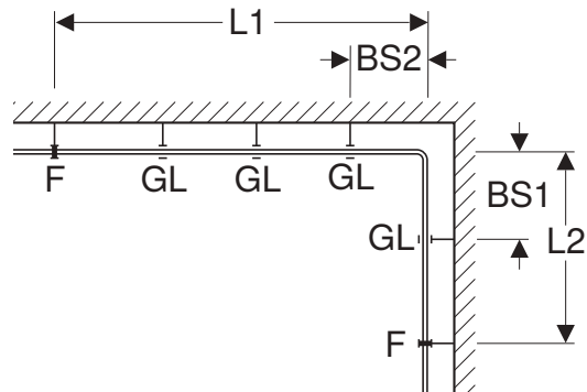
Abbildung 75: Dehnungsausgleich durch Richtungsänderung
