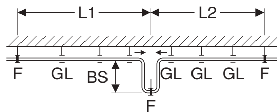
Abbildung 76: Dehnungsausgleich durch U-Bogen
