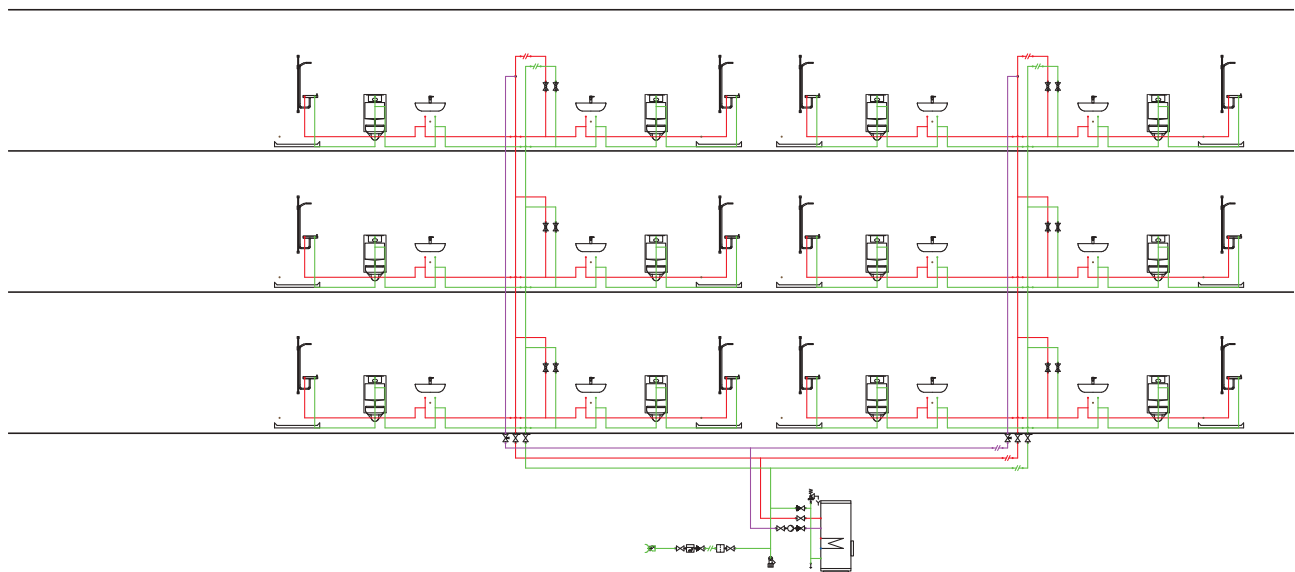
Abbildung 47: Vertikales Verteilkonzept mit mittiger Einspeisung
