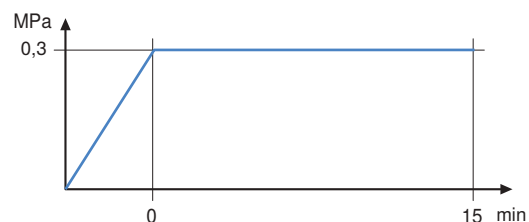
Abbildung 92: Prüfung „unverpresst undicht“, Schritt 1
