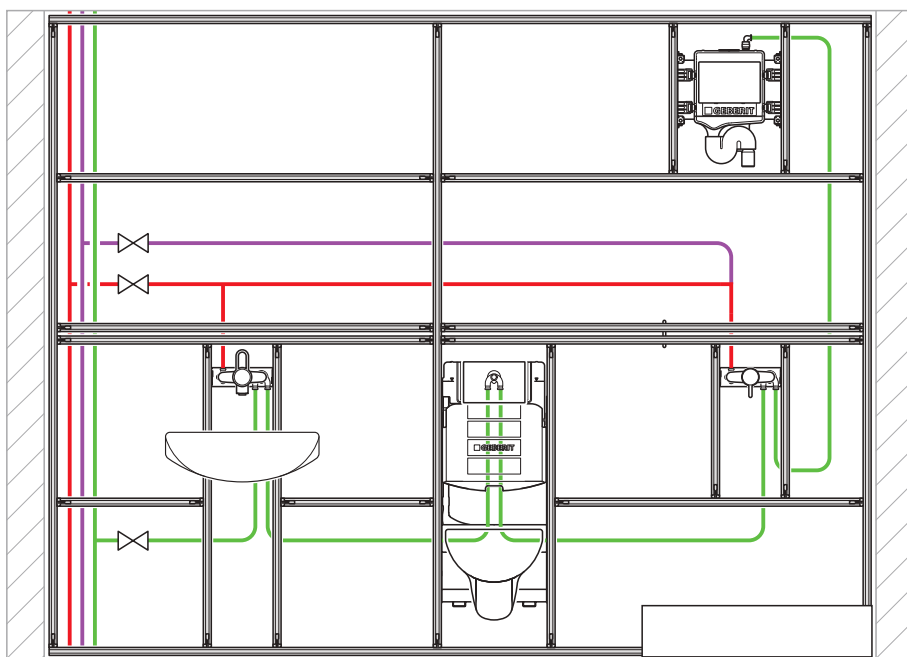
Abbildung 35: Beispiel Schema Hotelbadezimmer
