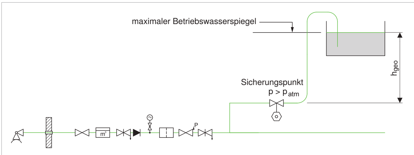
Abbildung 43: Bewertung des Sicherungspunktes
