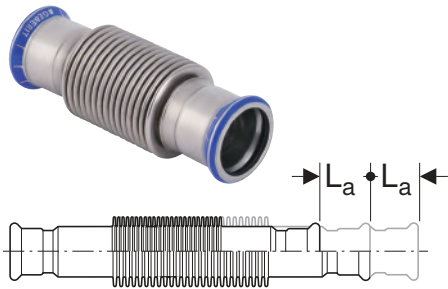
Abbildung 77: Geberit Mapress Edelstahl Axialkompensator
