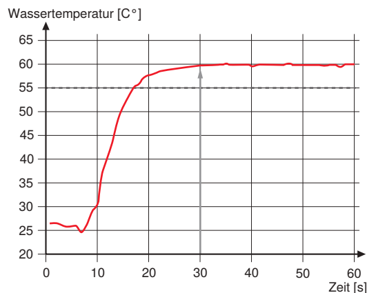
Abbildung 41: Typischer Temperaturverlauf von Warmwasser an einer Entnahmestelle
