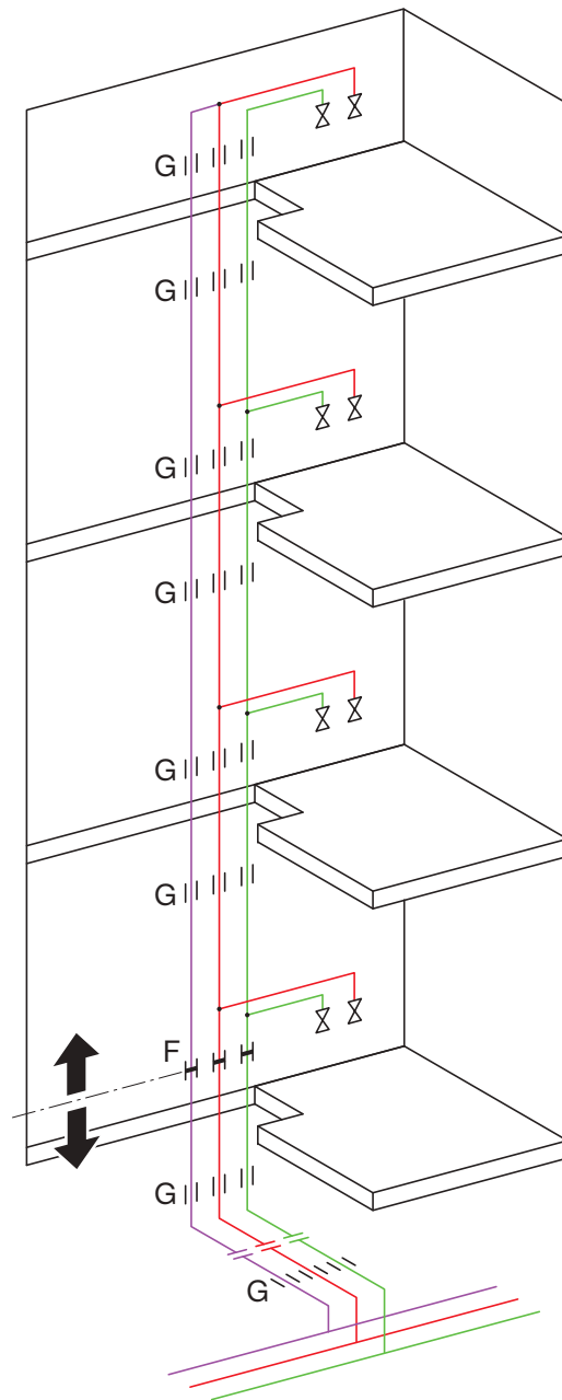
Abbildung 78: Steuerung der Längendeckung mit Fixpunkt im untersten Stockwerk
