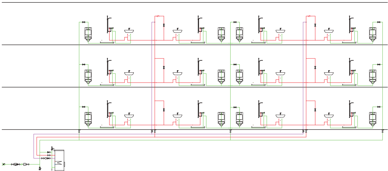
Abbildung 48: Vertikales Verteilkonzept mit separaten Schächten
