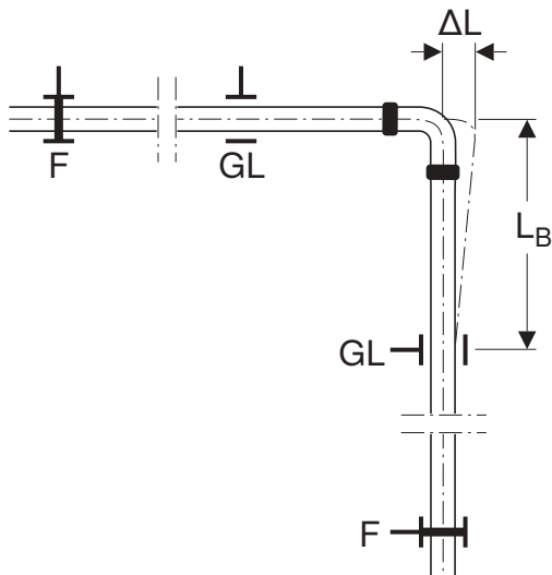
Abbildung 81: Dehnungsausgleich bei Richtungsänderung
