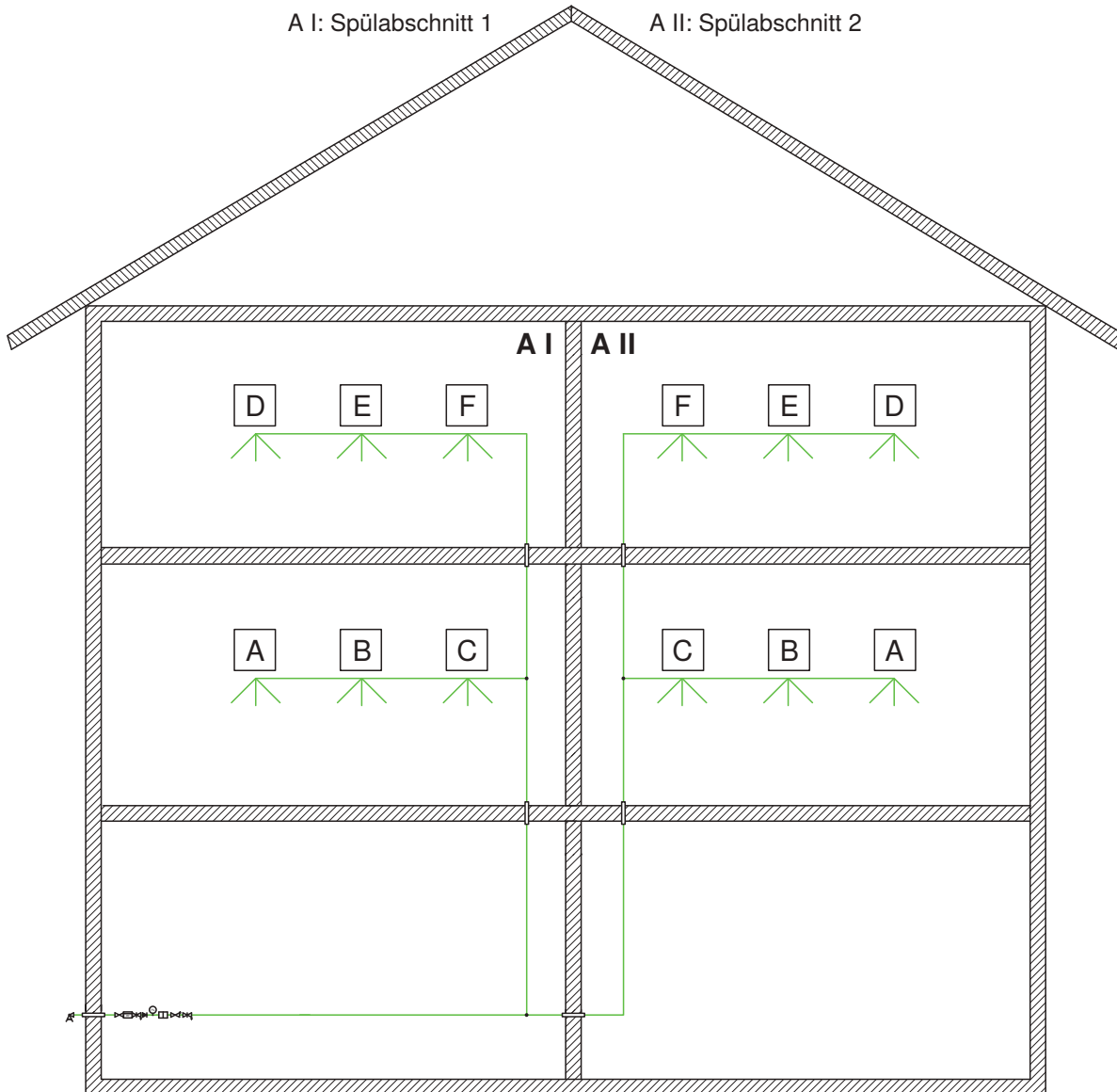
Abbildung 97: Spülabschnitte und Spülreihenfolge
