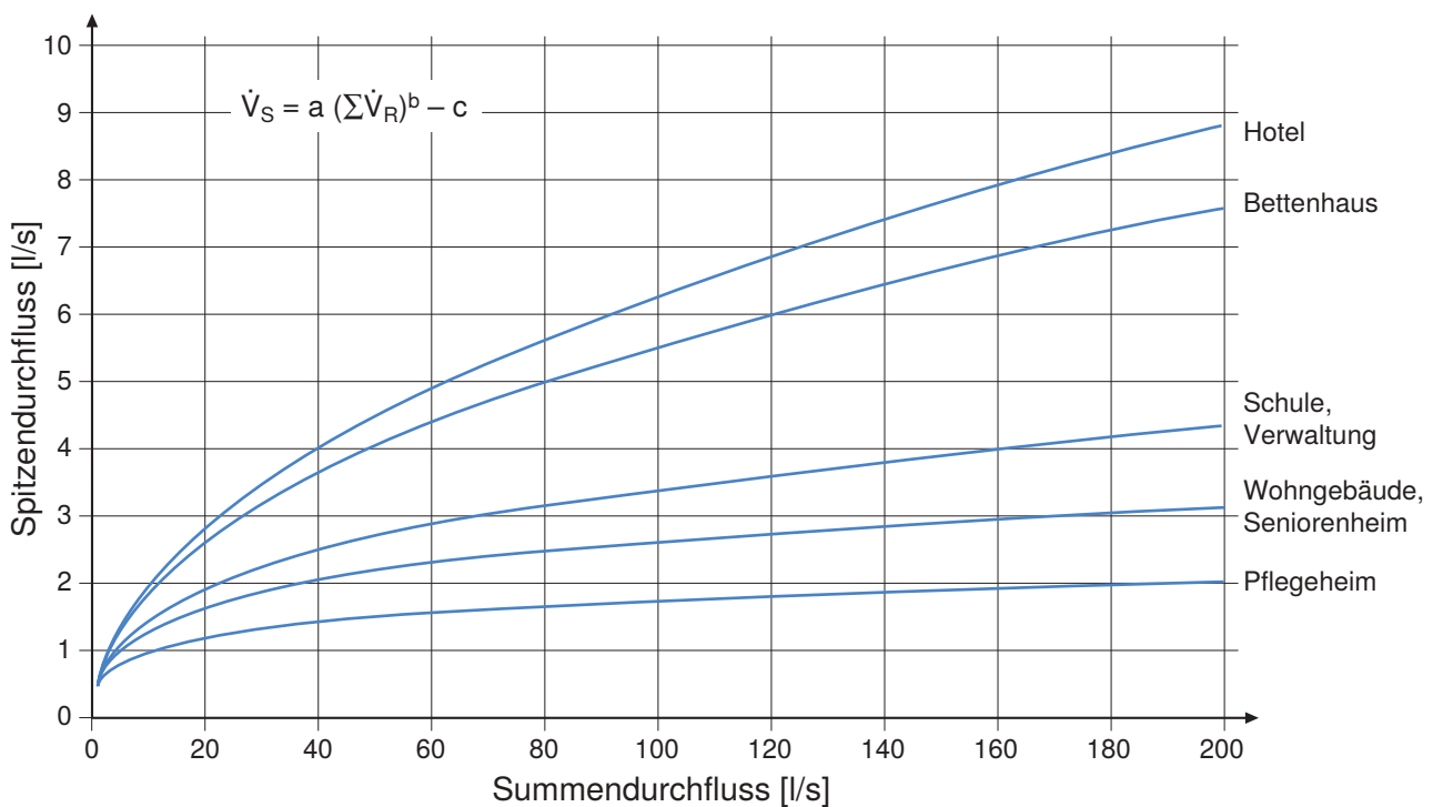
Abbildung 71: Grafische Darstellung der Spitzendurchflüsse
