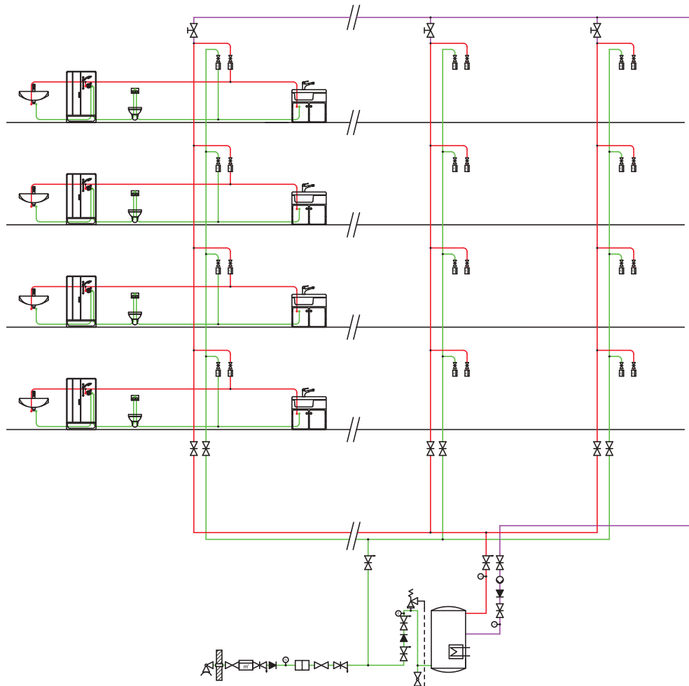
Abbildung 52: Obenliegender Zirkulationssammler mit separat geführtem Strang
