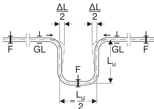
Abbildung 83: U-Bogen, aus Rohr gebogen
