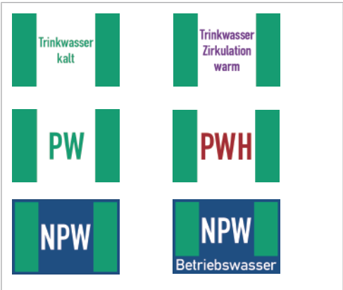
Abbildung 87: Beispiele für Rohrleitungskennzeichnungen gemäß DIN 2403
