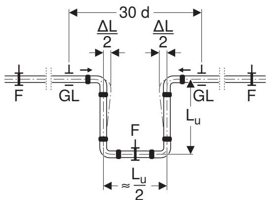
Abbildung 84: U-Bogen, mit Fittings hergestellt
