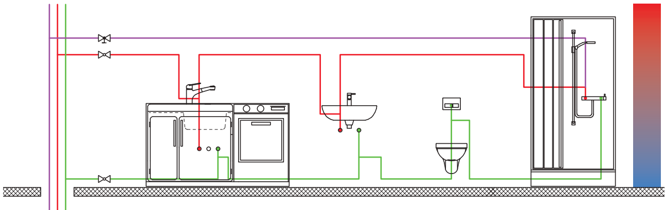
Abbildung 63: Temperatschichtung in einer Vorwand mit thermisch entkoppelter Leitungsführung
