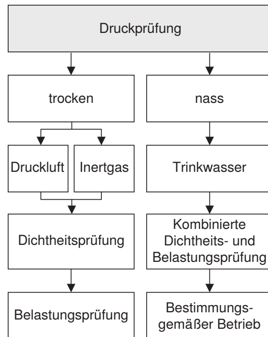
Abbildung 89: Möglichkeiten der Dichtheitsprüfung
