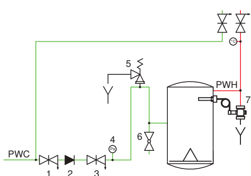
Direkt beheizt
