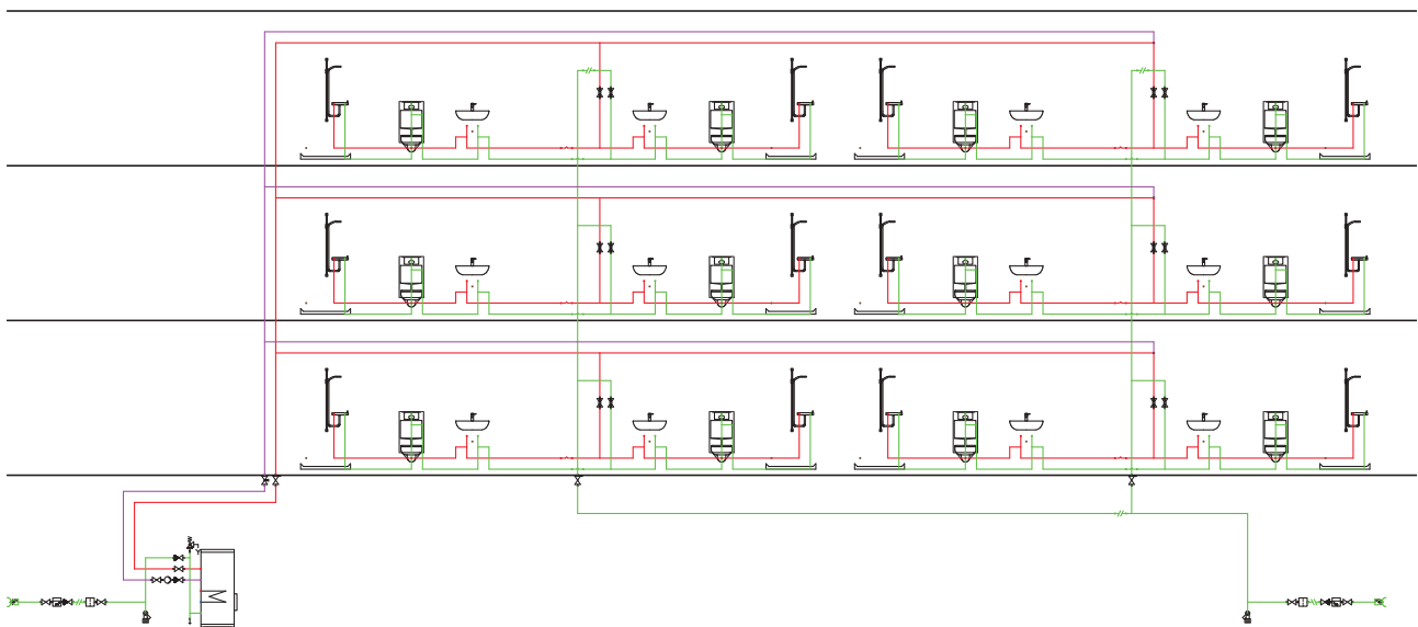
Abbildung 51: Horizontale und vertikale Verteilung mit zwei räumlich getrennten Hausanschlüssen
