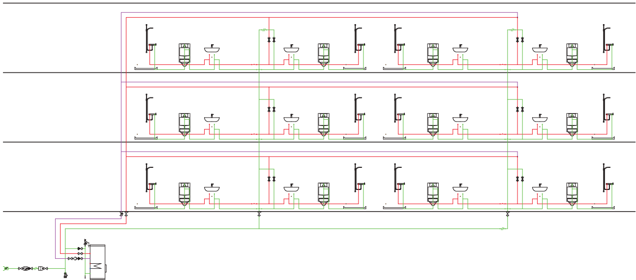
Abbildung 50: Horizontale und vertikale Verteilung mit einem Hausanschluss
