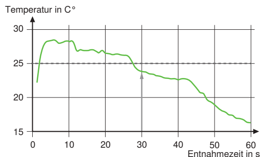
Abbildung 40: Beispielhafter Temperaturverlauf von Kaltwasser an einer Entnahmestelle
