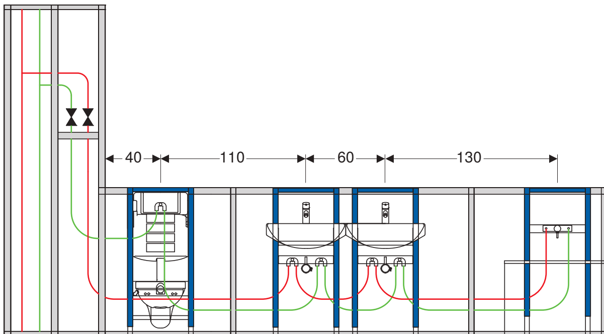
Abbildung 68: Durchgeschleifte Stockwerksinstallation mit Doppelanschlusswinkel
