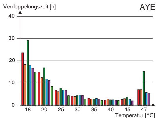
Abbildung 25: Verdoppelungszeit verschiedener Legionellenstämme in Abhängigkeit der Temperatur im Nährmedium AYE
