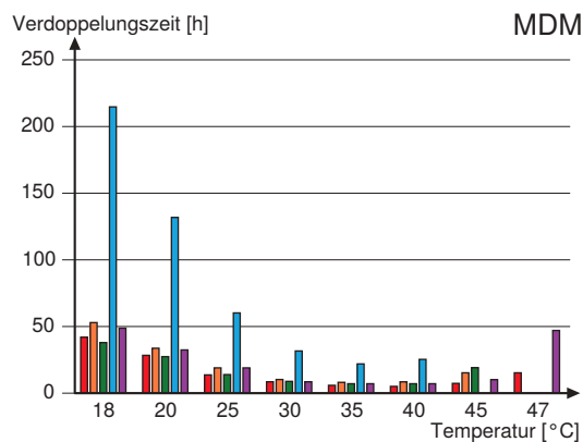
Abbildung 26: Verdoppelungszeit verschiedener Legionellenstämme in Abhängigkeit der Temperatur im Nährmedium MDM
