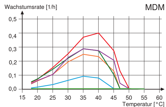
Abbildung 28: Umkehrwerte der Wachstumsraten verschiedener Legionellenstämme in Abhängigkeit der Temperatur im Nährmedium MDM
