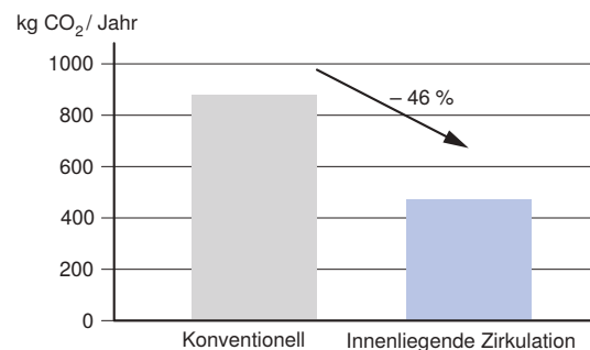
Abbildung 56: Vergleich CO 2 -Emission (CO 2 Emissionsfaktor Strommix 434 g/kWh)
