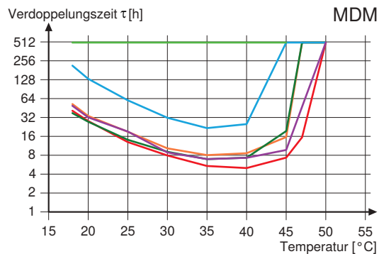
Abbildung 30: Logarithmische Darstellung der Verdoppelungszeit verschiedener Legionellenstämme in Abhängigkeit der Temperatur im Nährmedium MDM
