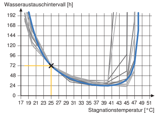
Abbildung 33: Wasseraustauschfunktion für die Medien AYE und MDM übereinandergelegt
