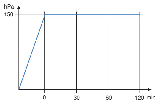
Abbildung 90: Dichtheitsprüfung mit ölfreier sauberer Druckluft oder Inertgas
