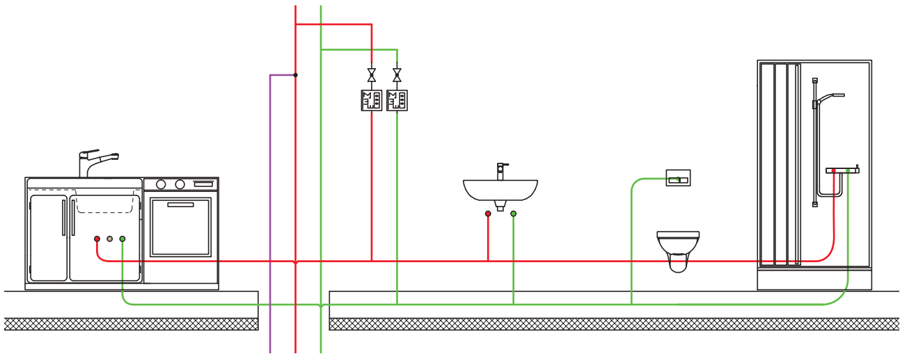
Abbildung 57: Stockwerksinstallation als T-Stück-Installation
