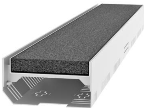
Steinrinne mit Entwässerungsschlitz 1-fach
