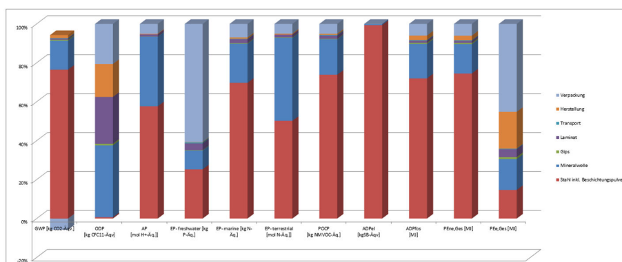
Abbildung 6: Prozentuale Anteile ausgewählter Komponenten, der Herstellung und der Transporte im Produktionsstadium anhand ausgewählter Umweltwirkungskategorien (Feuer- und Rauchschutztor El2120)
