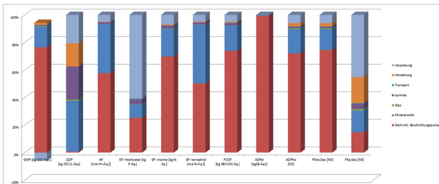
Abbildung 4: Prozentuale Anteile ausgewählter Komponenten, der Herstellung und der Transporte im Produktionsstadium anhand ausgewählter Umweltwirkungskategorien (Feuer- und Rauchschutztor El230)
