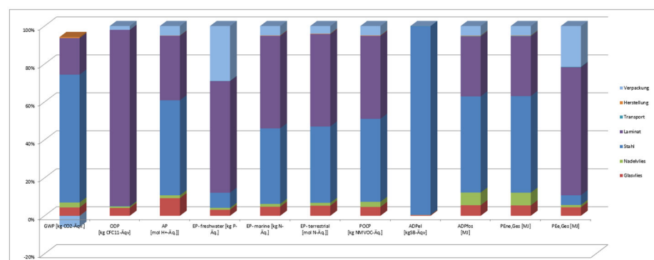
Abbildung 6: Prozentuale Anteile ausgewählter Komponenten, der Herstellung und der Transporte im Produktionsstadium anhand ausgewählter Umweltwirkungskategorien (Feuer- und Rauchschutzvorhang EI-60)
