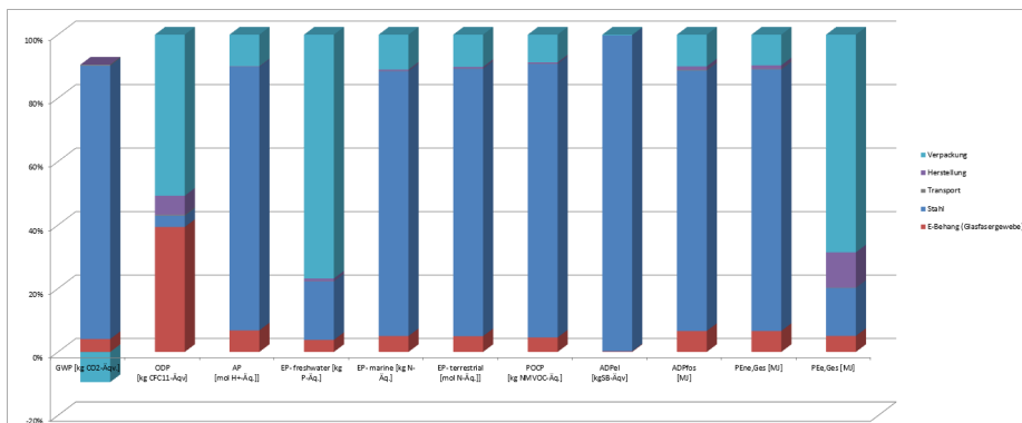
Abbildung 4: Prozentuale Anteile ausgewählter Komponenten, der Herstellung und der Transporte im Produktionsstadium anhand ausgewählter Umweltwirkungskategorien (Feuer- und Rauchschutzvorhang E-120)
