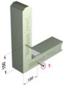
Einfachverschraubung Randabstand 150mm vom Riegelanfang
