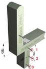
zusätzlicher Stützklotz ab 120mm Ausladung
