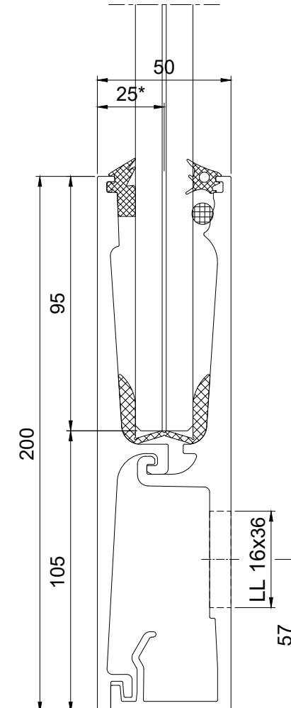
Abschlussblech 200x50x2
