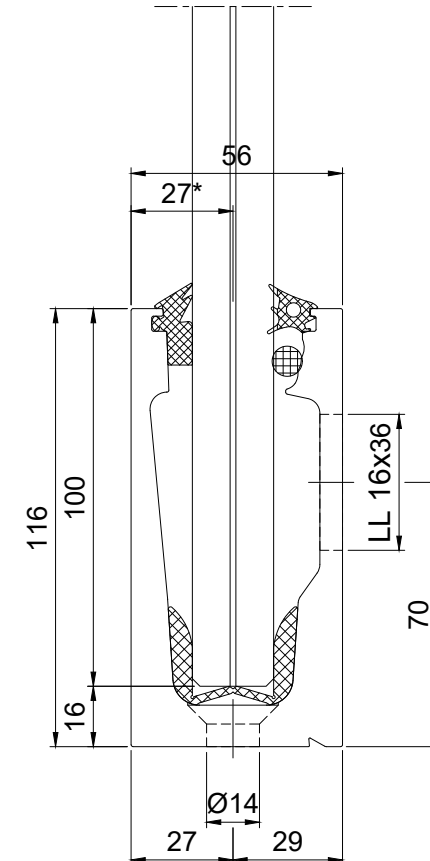
Abschlussblech 116x56x2
