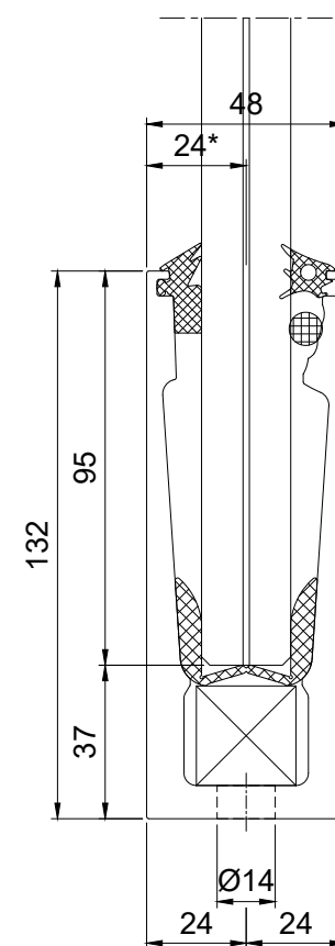
Abschlussblech 132x48x2
