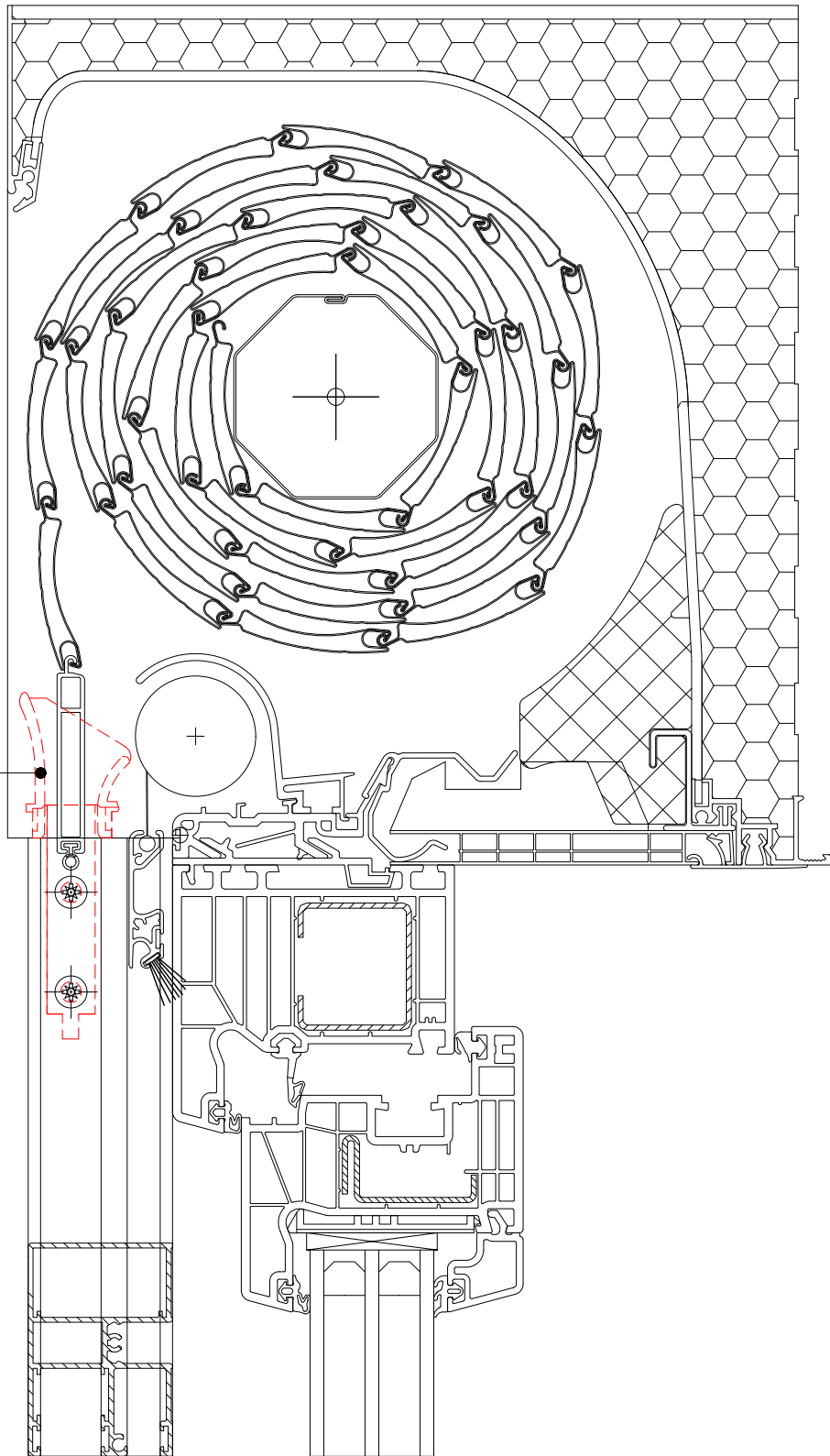
universale Einlaufhilfe Einlauftrichter
