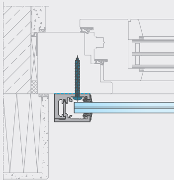
Holz-Fenster
