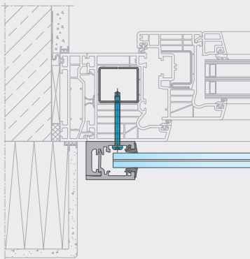
Kunststoff-Fenster
