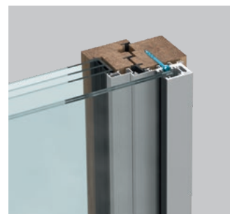
Holz-Alu-Fenster
