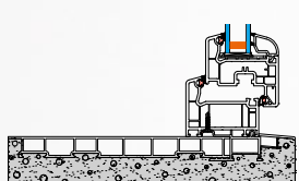
Ausführung B: betonierte Wände
