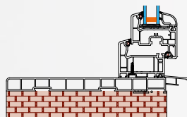
Ausführung A: Mauerwerk
