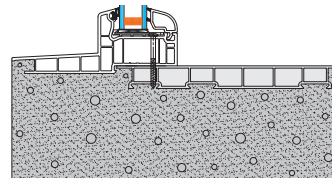
Typ 1, Ausführung B: betonierte Wände
