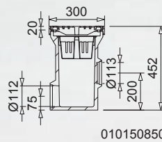
MEAGARD Hofablauf mit Gussrost (Abmessungen in mm)
