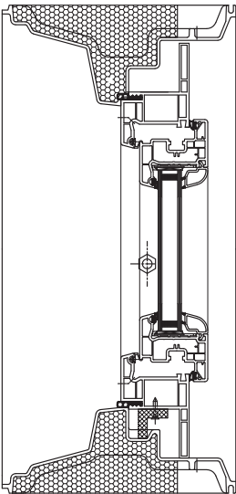
Querschnitt Renovierungsfenster für Zarge MEALUXIT Baujahr 1992 – 2005
