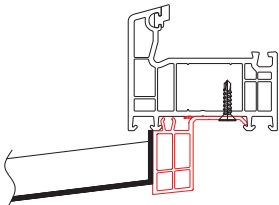
Fensterbankanschluss, Einbaubeispiel
