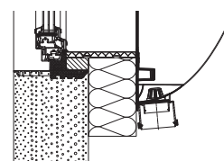
Überdämmte Ausführung von Perimeter-Abdeckrahmen MEAFIX ISO und Montagedämmplatte MEAFIX PRO
