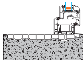
Typ 2, Ausführung B: betonierte Wände
