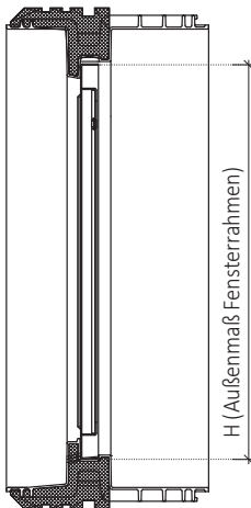
Querschnitt Zarge MEALUXIT mit Stahlfenstereinsatz
