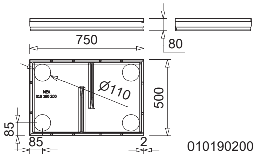
MEAGARD Fußabstreiferkasten, Abmessungen in mm
