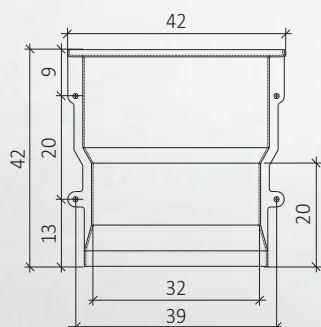
Abmessungen Lüftungsschacht (in cm)
