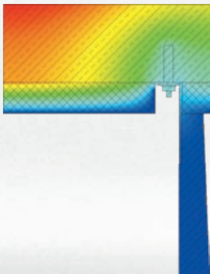
Befestigung mit örtlicher Dämmung
