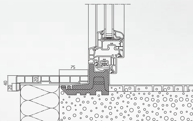
Querschnitt Zarge MEALUXIT mit Perimeter-Abdeckrahmen MEAFRAME (Abmessungen in mm)
