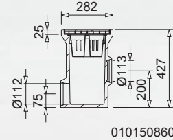
MEAGARD Hofablauf inkl. Maschenrost 30/20 vz, überdeckend, PKW-be-fahrbar (Abmessungen in mm)
