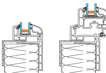
Typ 5 Festverglasung
