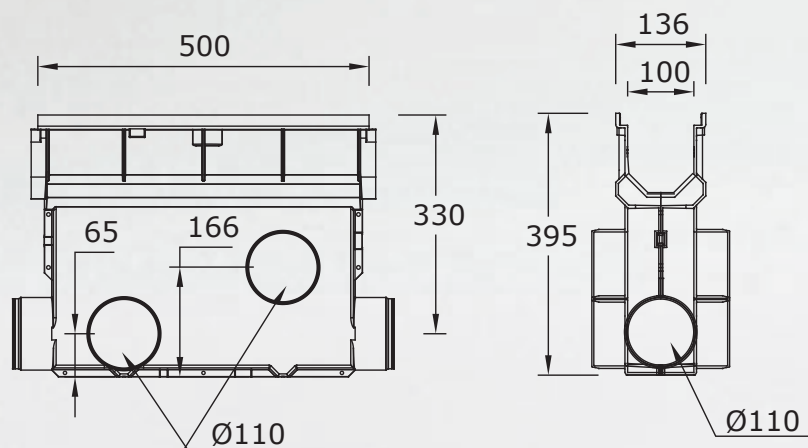
MEAFLUID Einlaufkasten, Abmessungen in mm
