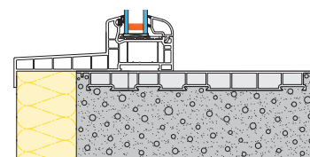
Typ 3, Ausführung B: betonierte Wände
