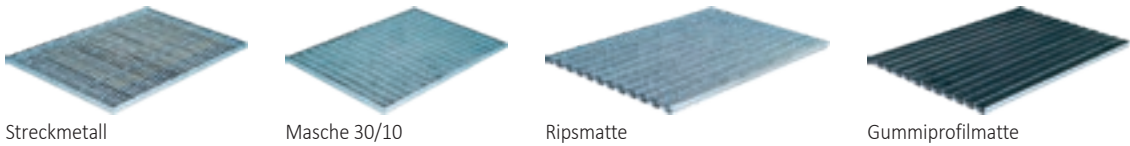
Abdeckungen für Fußabstreiferkästen
