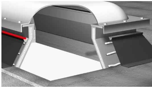
Versiegelung Verbundblech an Lichtkuppeln
