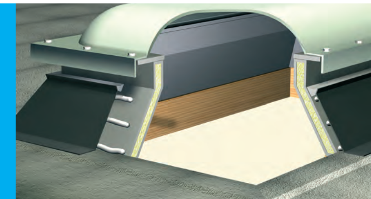
Anwendungsbeispiel: Wolfin Verbundbleche beim Lichtkuppelanschluss
