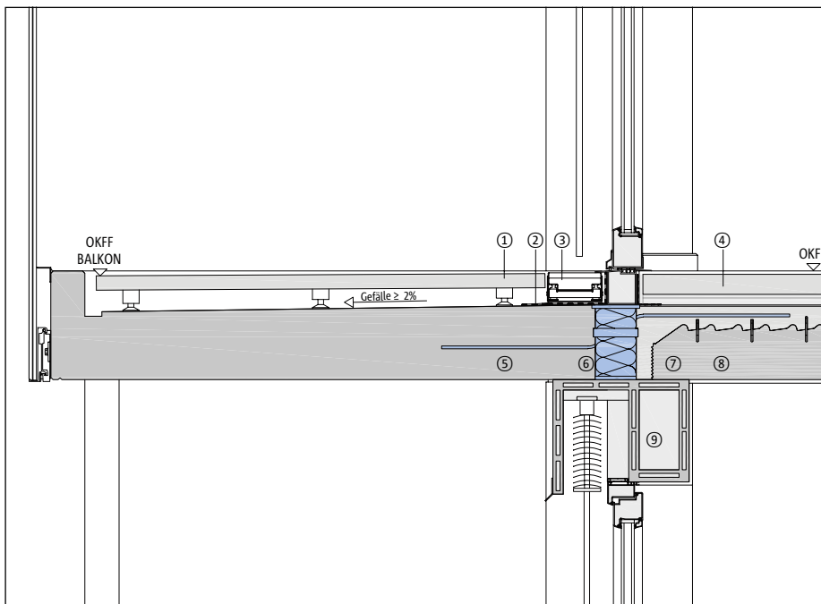
Anschluss gestützter Fertigteilbalkon an Stahlbetondecke zur nachträglichen Montage
