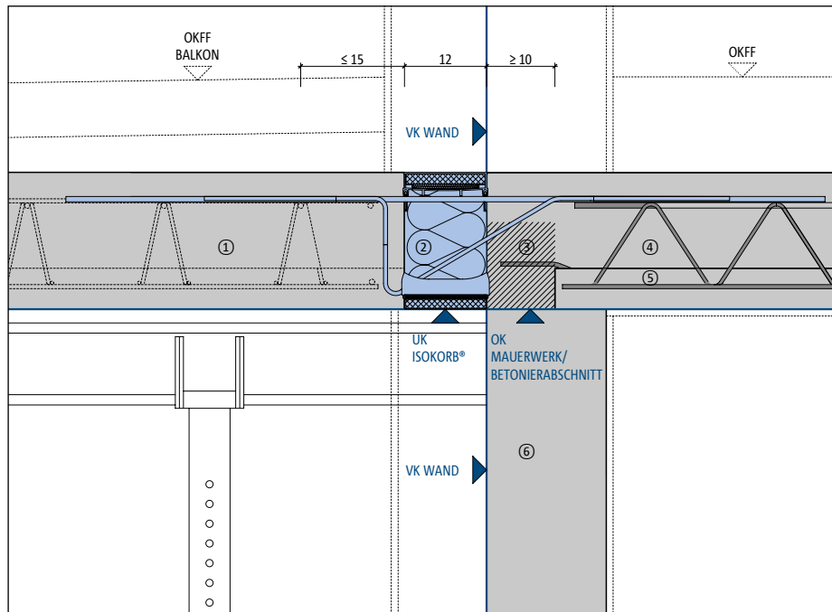
Form- und druckschlüssiger Einbau Schöck Isokorb®
