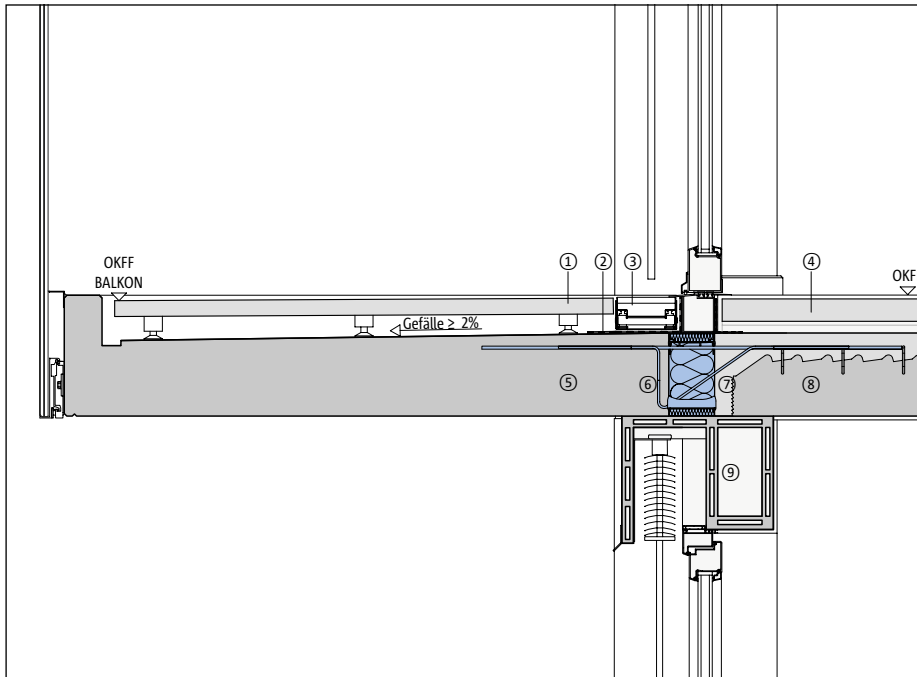
Anschluss frei ausragender Fertigteilbalkon an Stahlbetondecke zur nachträglichen Montage
