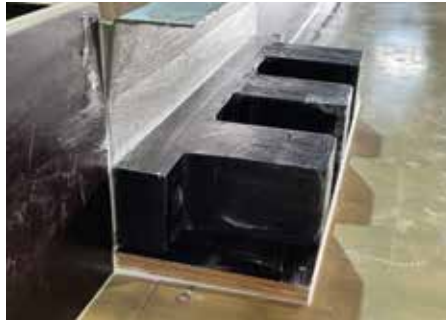
Abb. 1: IQ K-B Montageset (Part MS) für Teilset Balkon mit Schalung im Fertigteilwerk verlegen
